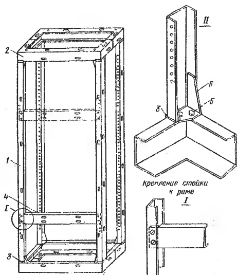
Рис. 8.2. Каркас объемный:
