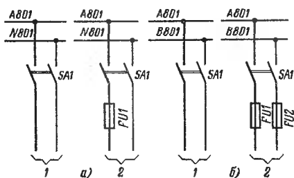
Рис. 6.23. Схема питания электроприемников, имеющих встроенные предохранители:
