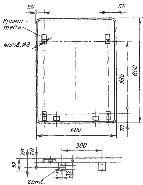
Рис. 8.17. Панель торцевая декоративная ПнТД-ЩПК
