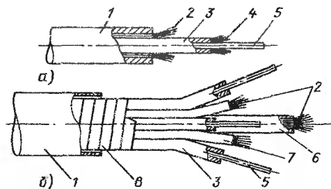
Рис. 11.4. Одно- (а) и четырехволоконный (б) оптические кабели:
