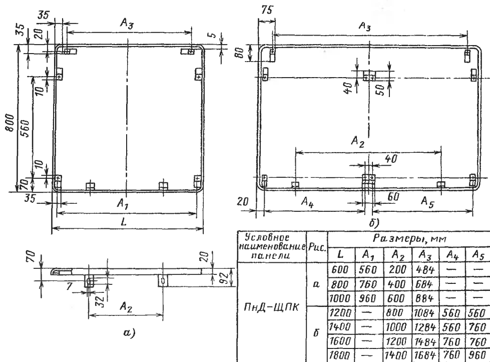
Рис. 8.16. Панель декоративная ПнД-ЩПК
