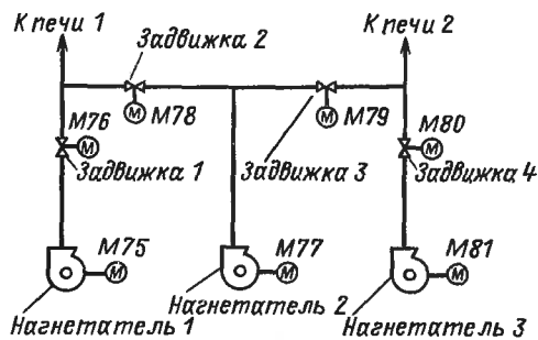
Рис. 4.6. Пример выполнения поясняющей технологической схемы
