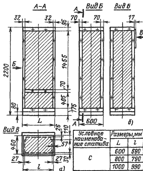
Рис. 8.27. Монтажные зоны статива С: а — исполнение I; б — исполнение II (остальное — см. рис. 8.27, а)
