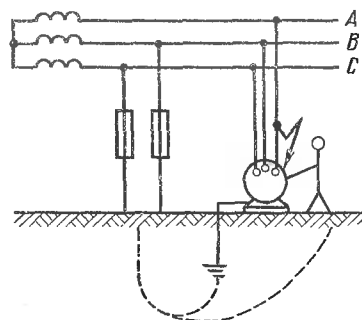
Рис. 14.1. Заземление электроприемника
