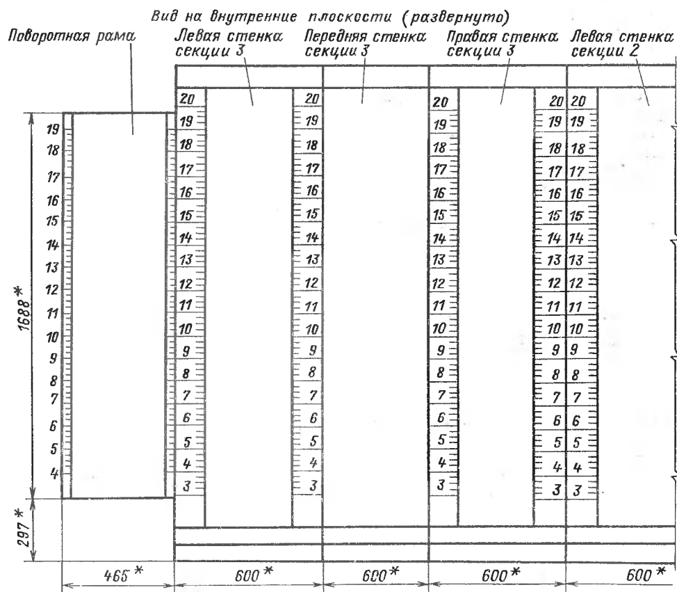
Рис. 9.19. Пример выполнения форматно-заготовок чертежа «Вид на внутренние плоскости» для многосекционного щита с поворотной рамой
