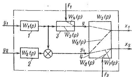
Рис. 18.1. Пример исходной алгоритмической структурной схемы объекта автоматизации
