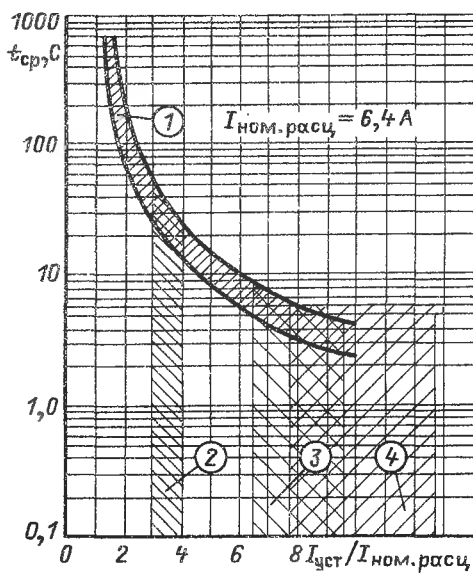
Рис. 6.8. Времятоковые характеристики автоматических выключателей серии АП50-3МТ на номинальный ток 6,4 А
