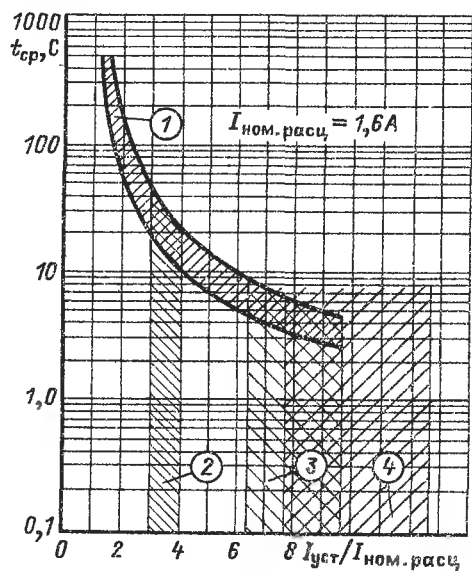
Рис. 6.5. Времятоковые характеристики автоматических выключателей серии АП50-3МТ на номинальный ток 1,6 А
