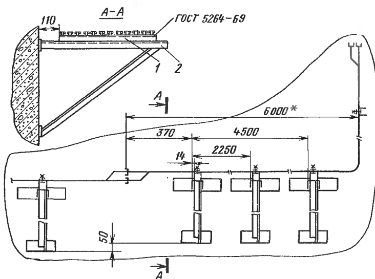
Рис. 12.22. Блок на швеллере угловой (установка на стене):
