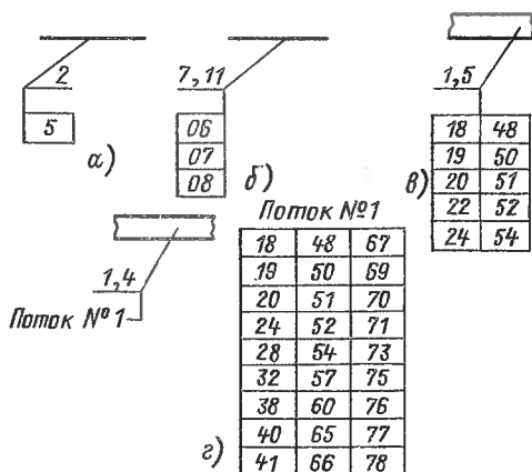
Рис. 13.20. Примеры нумерации электрических и трубных проводок:
