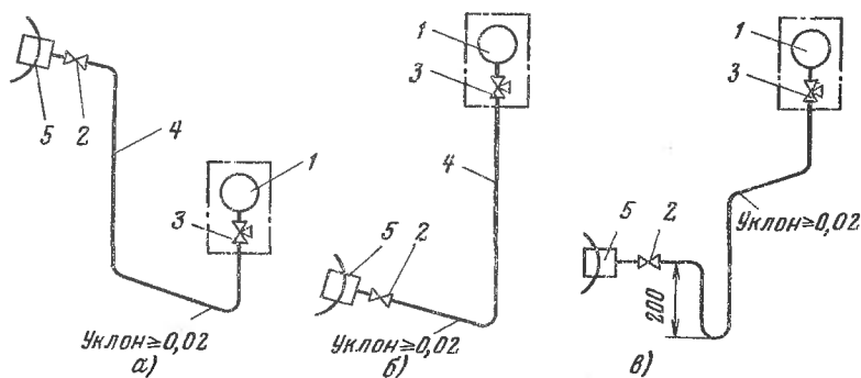
Рис. 12.1. Схемы импульсных трубных проводок для измерения давления жидкости и пара: а — манометр установлен ниже места отбора давления (жидкость и пар); б — то же выше места отбора давления (жидкость); в — то же выше места отбора давления (пар); 1 — манометр; 2 — запорный вентиль; 3 — трехходовой кран; 4 — импульсная труба; 5 — отбор давления
