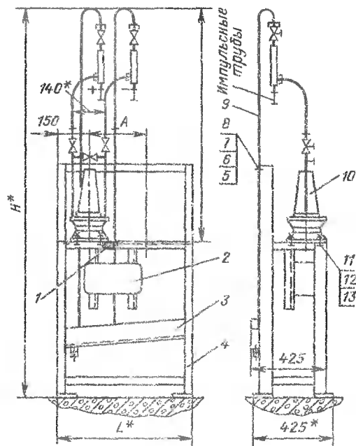
Рис. 17.11. Пример групповой установки дифманометров мембранных ДМ по
