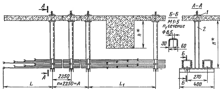
Рис. 12.21. Блок на обойме прямой (установка на потолочном перекрытии):
