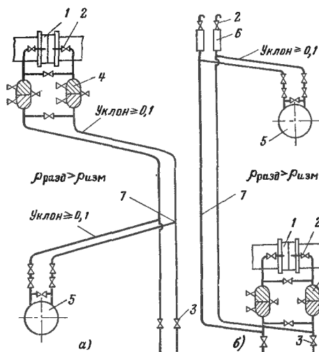
Рис. 12.12. Схемы для измерения расхода агрессивной жидкости при \rho_{разд} > \rho_{изм} :
