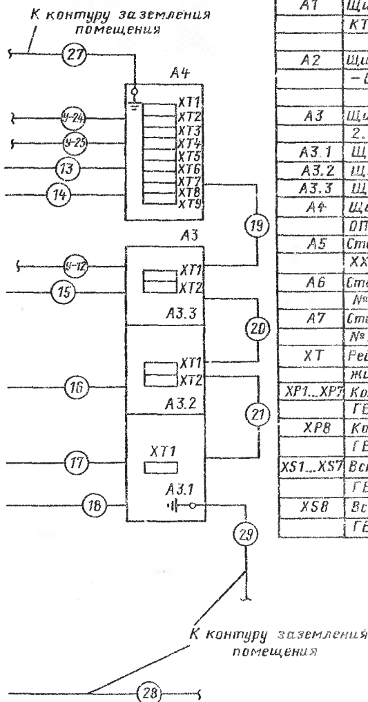
Рис. 9.23. Пример выполнения схемы электрических соединений КТС ОП
