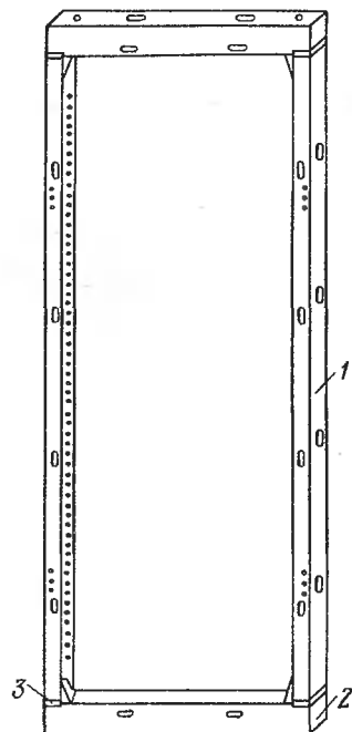
Рис. 8.3. Каркас плоский:
