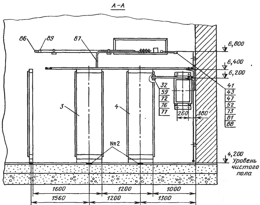
Рис. 9.21. Разрез А-А к рис. 9.20
