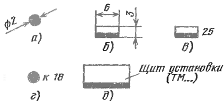
Рис. 13.19. Условные графические изображения приборов, щитов и пультов:
