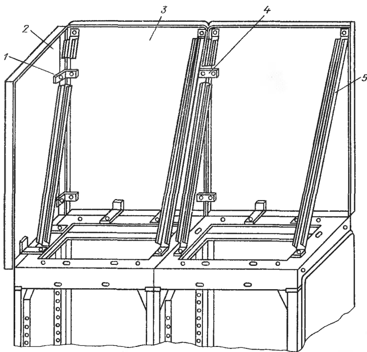
Рис. 8.20. Установка панелей ПнД-ЩПК и ПнТД-ЩПК на каркасах объемных щитов: 1 — угольник; 2 — панель ПнД-ЩПК; 3 — панель ПнД-ЩПК; 4 — пластина; 5 — кронштейн
