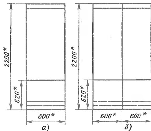
Рис. 9.17. Примеры выполнения форматно-заготовок чертежа «Вид спереди»: а — для шкафного щита; б — для двухсекционного щита
