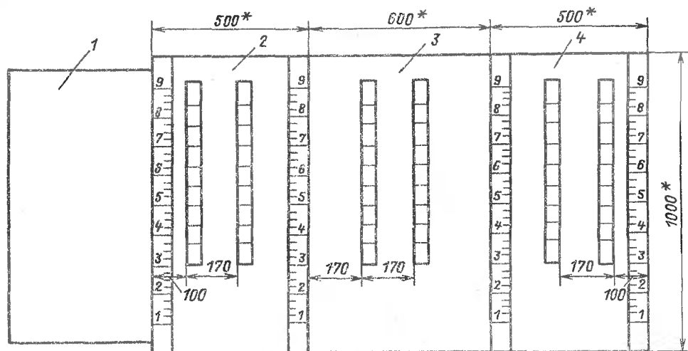
Рис. 13.29. Расположение блоков зажимов в щите ЩШМ при вводе проводов снизу: а — щит 600 × 500 × 100 мм; б — щит 400 × 500 × 600 мм; 1 — дверь; 2 — левая стенка; 3 — передняя стенка; 4 — правая стенка
