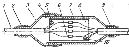
Рис. 11.13. Соединение многоволоконных ОК с помощью цилиндрической муфты:
