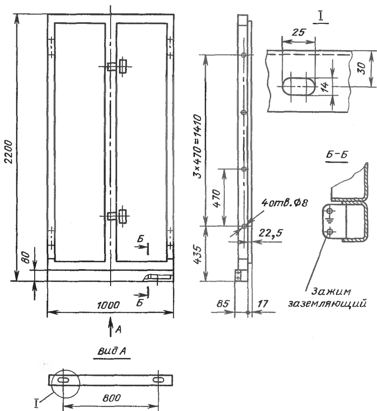
Рис. 8.14. Панель вспомогательная с дверью ПнВ-Д
