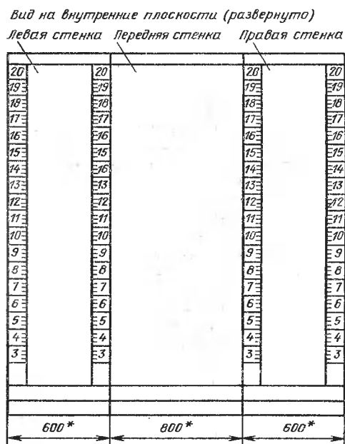
Рис. 9.18. Пример выполнения форматно-заготовок для чертежа «Вид на внутренние плоскости» для шкафного щита
