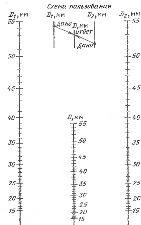
Рис. 11.3. Номограмма для определения внутреннего диаметра защитной трубы для прокладки проводников двух различных диаметров при общем числе их более двух
