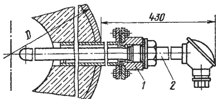
Рис. 17.3. Установка термоэлектрического термометра в опрессовке фланцевой с бобышкой на трубопроводе ( D = 530 мм) или металлической стенке с внутренней кирпичной кладкой по ТМ4-153—75:
