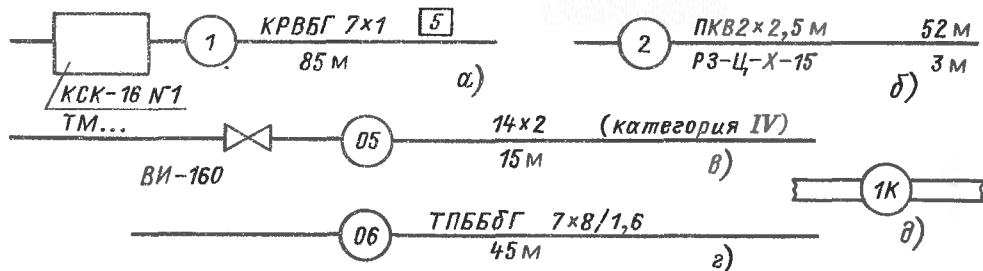
Рис. 13.9. Изображения внешних проводок:
