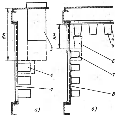
Рис. 8.42. Пример определения «теней» от прибора или аппаратов:
