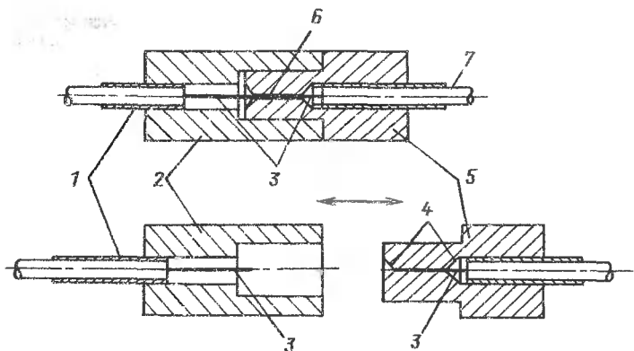
Рис. 11.9. Разъемный соединитель многократного действия для соединения ОВ с пластмассовым покрытием:
