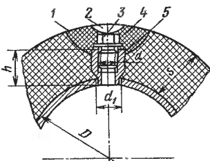
Рис. 17.2. Закладная конструкция ЗК4-1—75:
