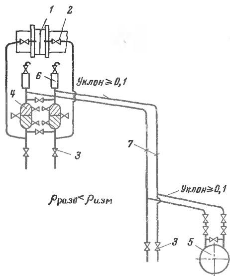
Рис. 12.14. Схема для измерения расхода агрессивной жидкости (дифманометр установлен ниже сужающего устройства) при P_{разд} < P_{изм} :
