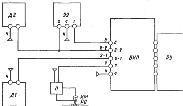
Рис. 5.6. Принципиальная пневматическая схема следящей автоматической системы регулирования:
