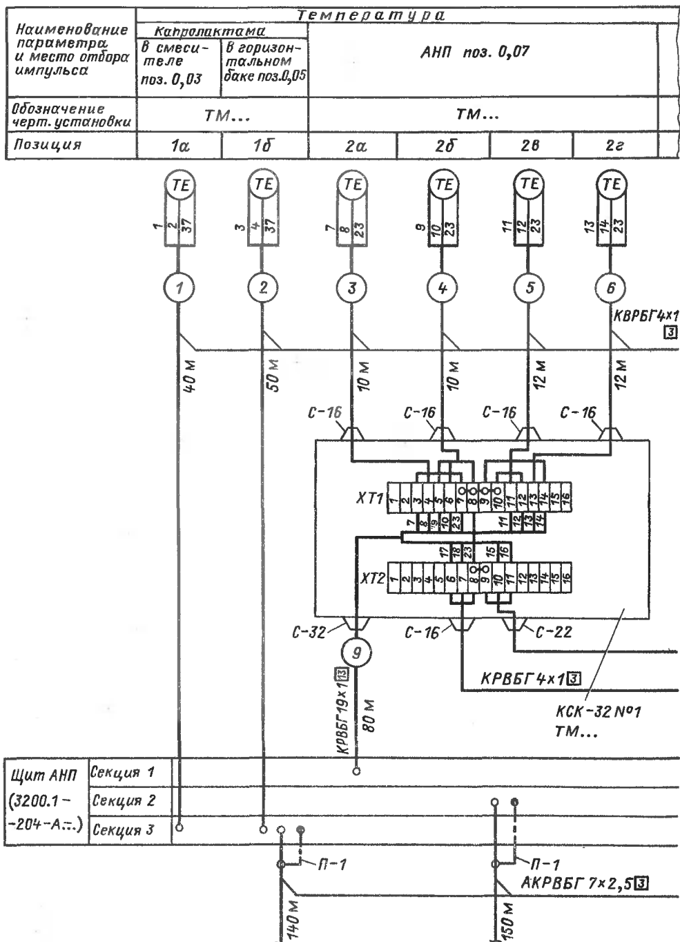
Рис. 13.6. Фрагмент схемы внешних проводов с применением кабелей контрольных и коробок соединительных
