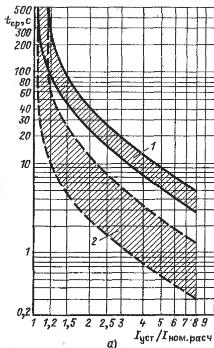
Рис. 6.15. Времятоковые характеристики тепловых реле типа ТРН:
