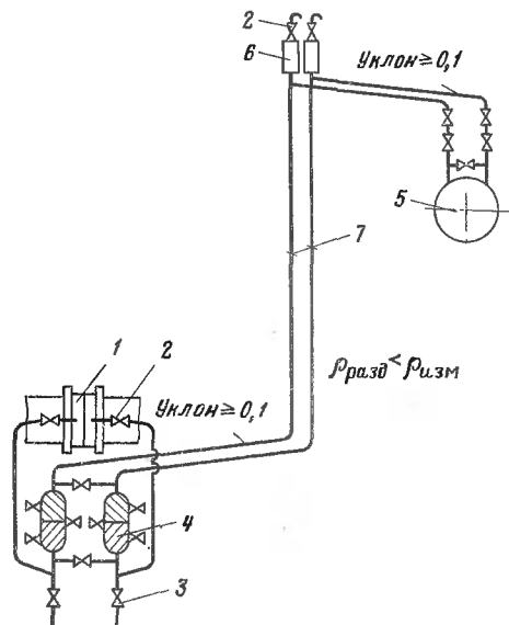
Рис. 12.13. Схемы для измерения расхода агрессивной жидкости (дифманометр установлен выше сужающего устройства) при \rho_{разд} < \rho_{изм} :
