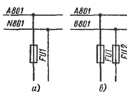
Рис. 6.21. Схема питания электроприемников, имеющих встроенные выключатели (смена предохранителей в данной схеме должна производиться при отключенном выключателе прибора):
