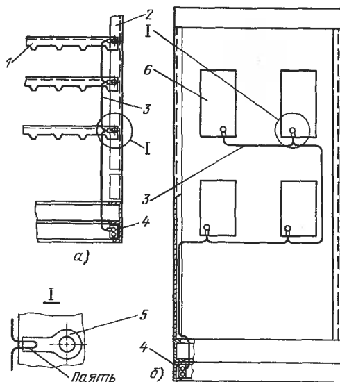
Рис. 8.22. Примеры выполнения зануления (заземления) угольников, скоб (а), приборов и аппаратов, имеющих зажим «Земля» (б): 1 — угольник У, УЗ (скоба С, СЗ); 2 — стойка щита, стativa; 3 — гибкий неразрезанный проводник; 4 — заземляющий зажим М6; 5 — кабельный наконечник; 6 — прибор (аппарат)
