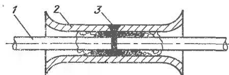
Рис. 11.12. Соединение ОВ с помощью втулок:
