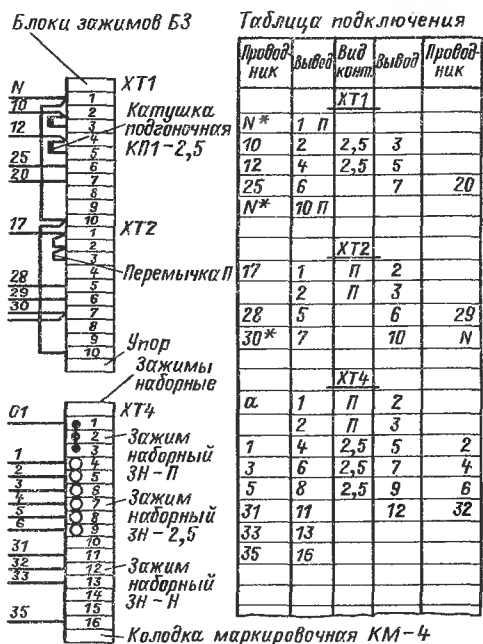
Рис. 9.16. Пример заполнения таблицы подключения для блоков зажимов с условными обозначениями зажимов с перемычкой и подгоночными катушками
