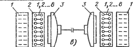
Рис. 9.28. Зажимно-модульные и межмодульные соединители комплекта «Ремиконт Р-100»
