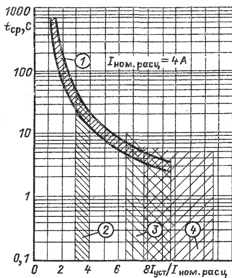
Рис. 6.7. Времятоковые характеристики автоматических выключателей серии АП50-3МТ на номинальный ток 4 А
