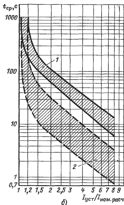
Рис. 6.15. Времятоковые характеристики тепловых реле типа ТРН:
