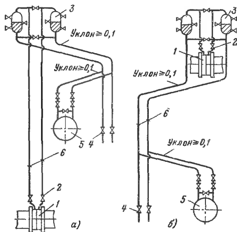
Рис. 12.15. Схемы для измерения расхода агрессивного газа при P_{разд} > P_{изм} :
