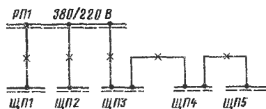
Рис. 6.3. Радиально-магистральная (смешанная) схема питающей сети
