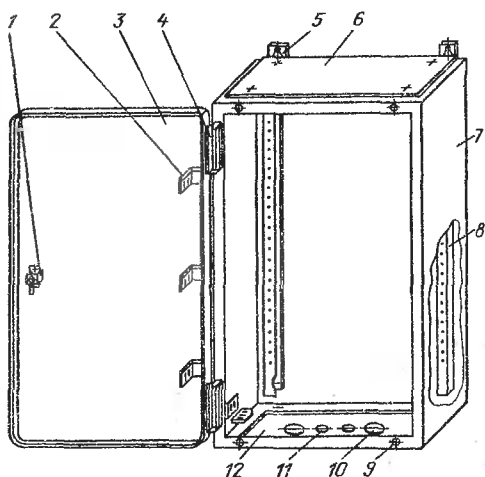
Рис. 8.10. Шкаф малогабаритный:
