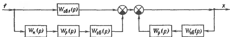
Рис. 18.6. Структурные схемы системы, представленной на рис. 18.5, по каналу возмущающего воздействия
