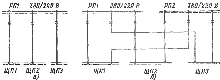
Рис. 6.2. Радиальные схемы питающей сети:
