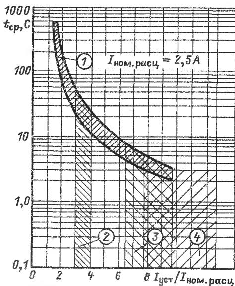
Рис. 6.6. Времятоковые характеристики автоматических выключателей серии АП50-3МТ на номинальный ток 2,5 А
