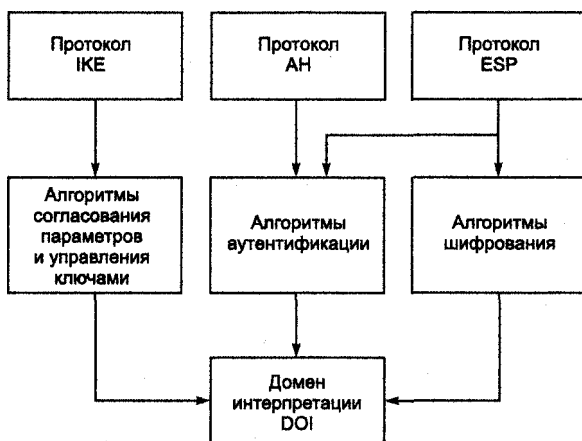
Рис. 12.2. Архитектура стека протоколов IPSec
