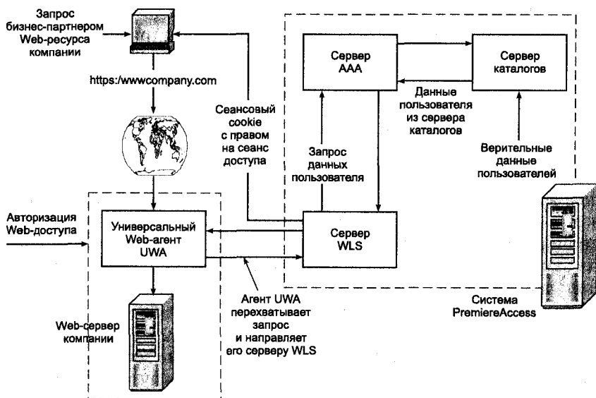
Рис. 13.3. Схема управления Web-доступом
