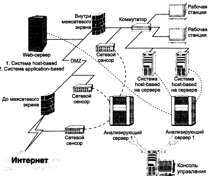
Рис. 14.5. Общая схема функционирования распределенной dIDS
