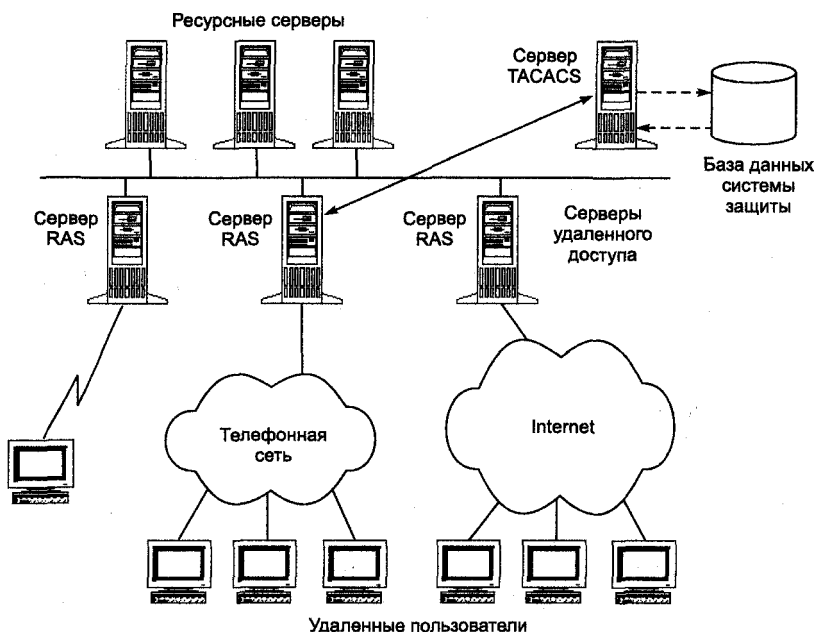
Рис. 13.5. Схема централизованного контроля удаленного доступа
