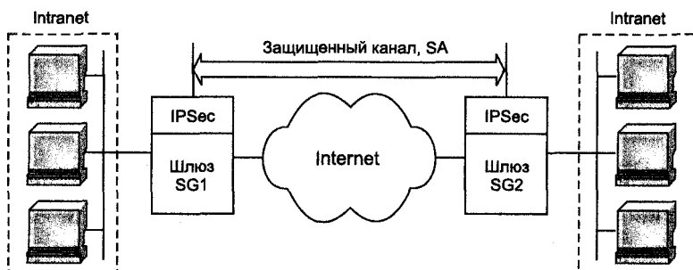
Рис. 12.9. Схема шлюз-шлюз
