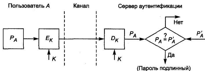
Рис. 7.1. Простая аутентификация с использованием пароля
