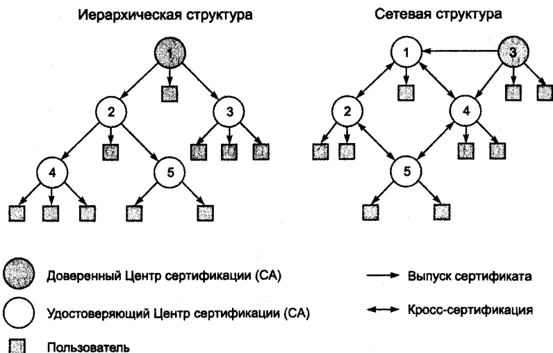
Рис. 13.10. Иерархическая и сетевая архитектуры систем управления сертификатами
