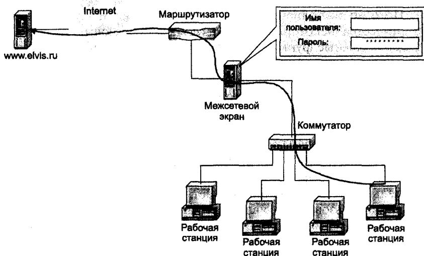
Рис. 9.3. Схема аутентификации пользователя по предъявляемому паролю
