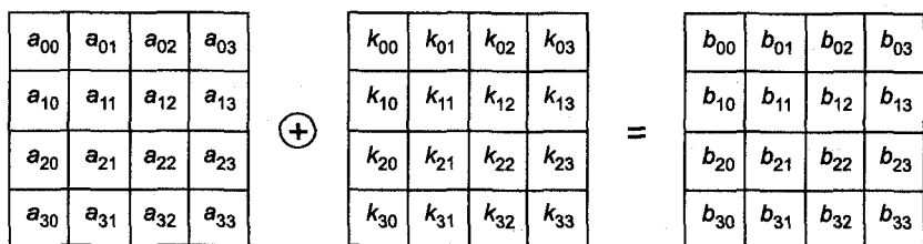
Рис. 6.8. Преобразование AK (AddRoundKey) производит сложение XOR каждого столбца массива State со словом из ключевого набора
