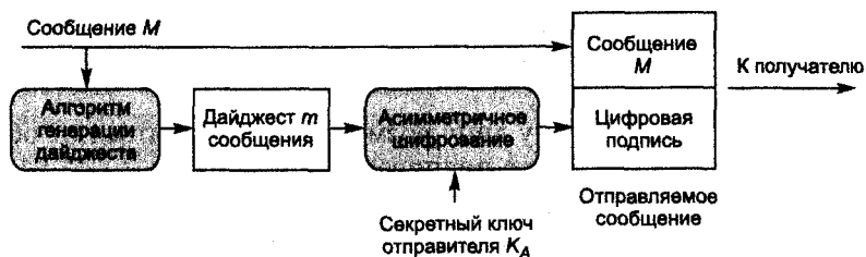
Рис. 5.6. Схема формирования электронной цифровой подписи
