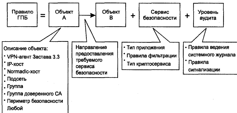
Рис. 16.1. Структура правила глобальной политики безопасности
