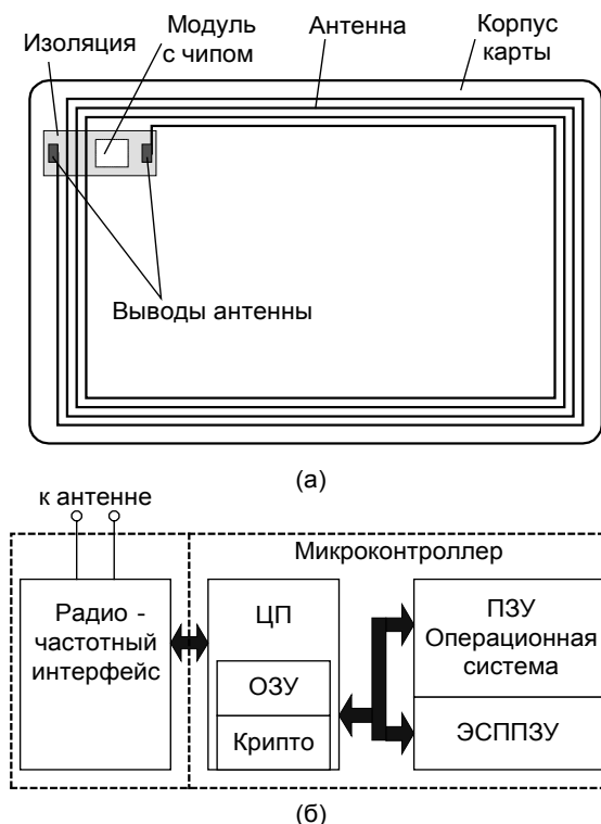
Рис. 5.5. Микропроцессорная смарт-карта с бесконтактным интерфейсом: а) конструктивные элементы бесконтактной смарт-карты; б) архитектура интегральной схемы (чипа) бесконтактной смарт-карты
