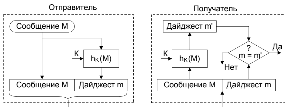
Рис. 5.7. Применение для аутентификации односторонней хэш-функции с параметром-ключом
