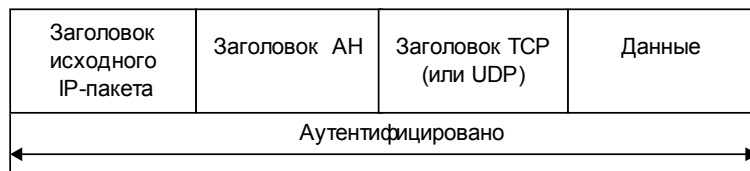
IP-пакет после применения протокола АН в туннельном режиме
