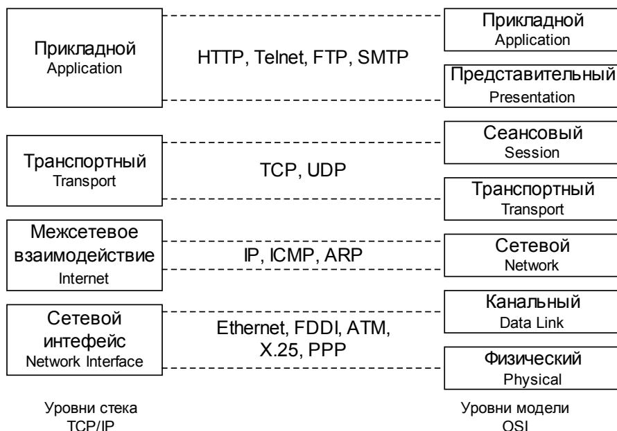
Рис. 8.1. Уровни стека протоколов TCP/IP
