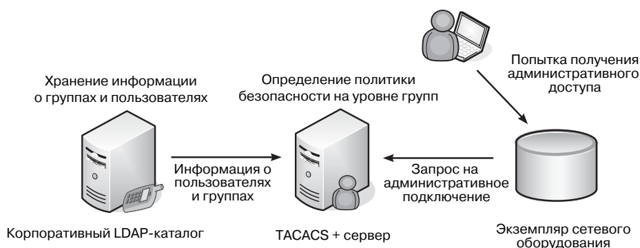
Рис. 14.1. Использование корпоративного LDAP-каталога для управления учетными записями
