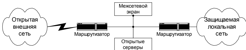
Рис. 9.10. Защита локальной сети с помощью МЭ с одним сетевым интерфейсом
