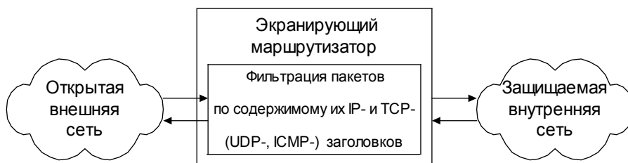
Рис. 9.6. Схема функционирования пакетного фильтра
