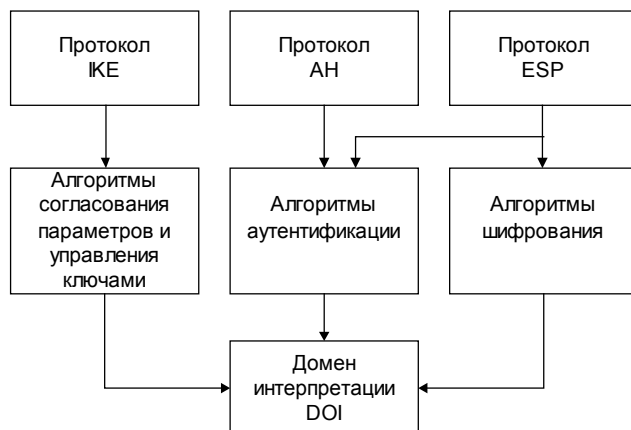
Рис. 8.11. Архитектура стека протоколов IPsec
