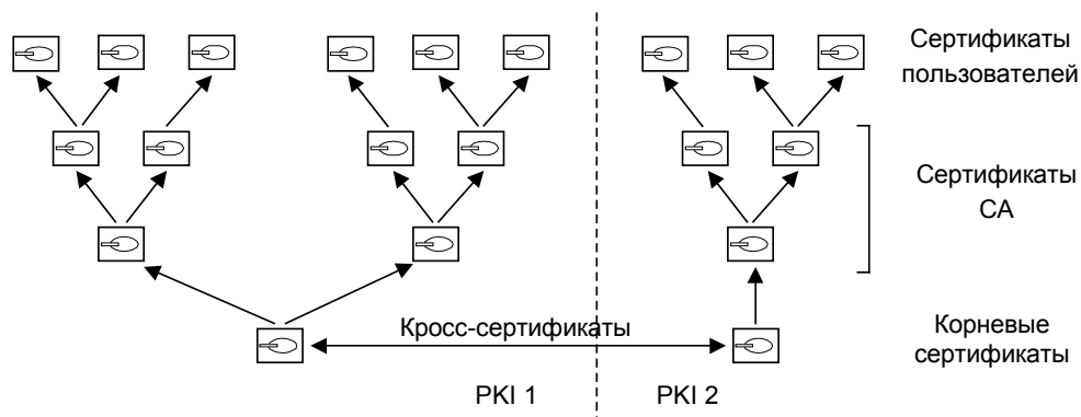
Рис. 4.28. Иерархическая структура сертификатов
