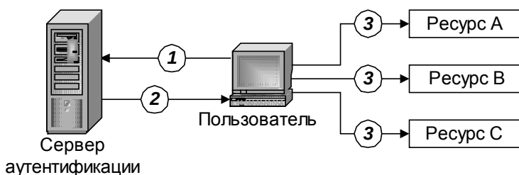
Рис. 5.9. Простое SSO-решение – автоматизация входа
