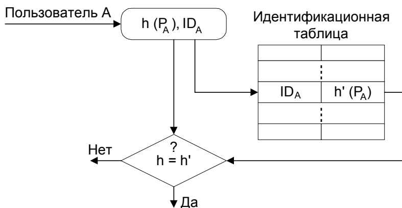
Рис. 5.2. Использование односторонней функции для проверки пароля
