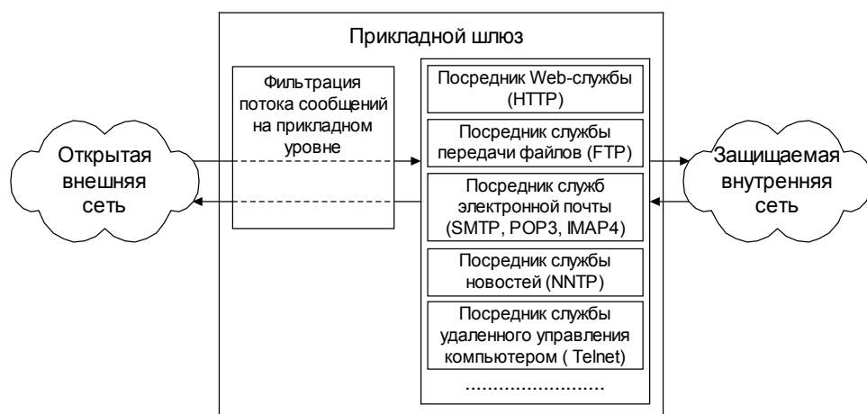
Рис. 9.8. Схема функционирования прикладного шлюза
