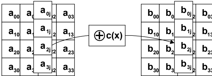
Рис. 4.11. Преобразование MC (MixColumn) поочередно обрабатывает столбцы массива State
