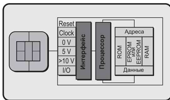
Рис. 5.4. Пример контактной микропроцессорной смарт-карты
