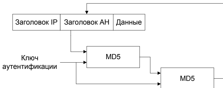
Рис. 8.16. Структура HMAC-алгоритма
