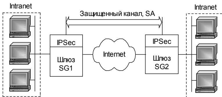
Рис. 8.18. Схема шлюз–шлюз
