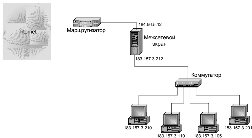
Рис. 9.4. Трансляция сетевых адресов
