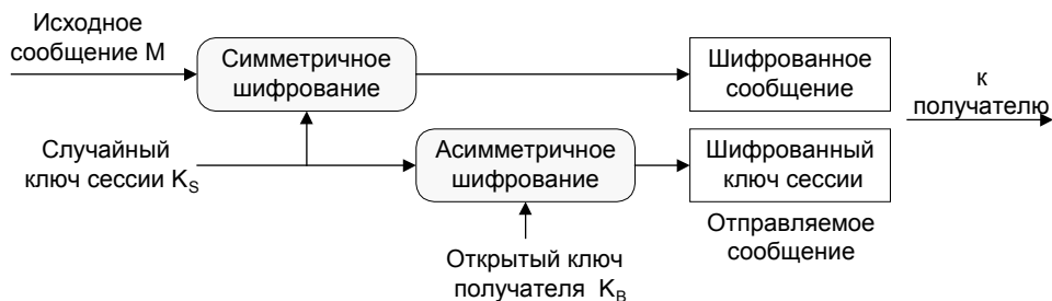
Рис. 4.24. Схема шифрования сообщения комбинированным методом
