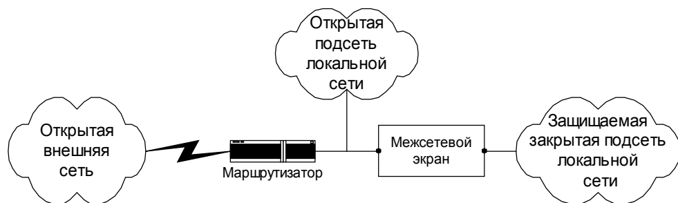
Рис. 9.12. Схема с защищаемой закрытой и не защищаемой открытой подсетями
