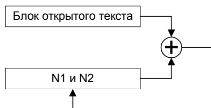
Рис. 4.8. Выработка гаммы шифра в режиме гаммирования с обратной связью
