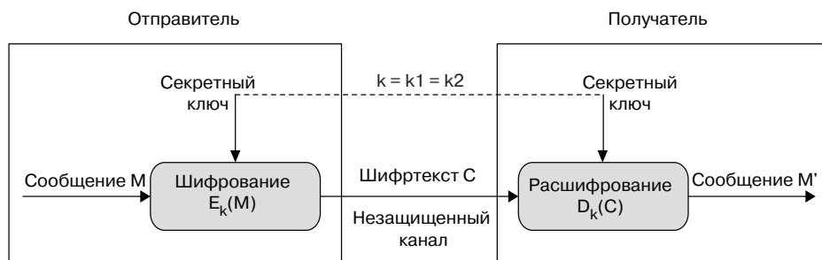
Рис. 4.3. Схема симметричной криптосистемы шифрования
