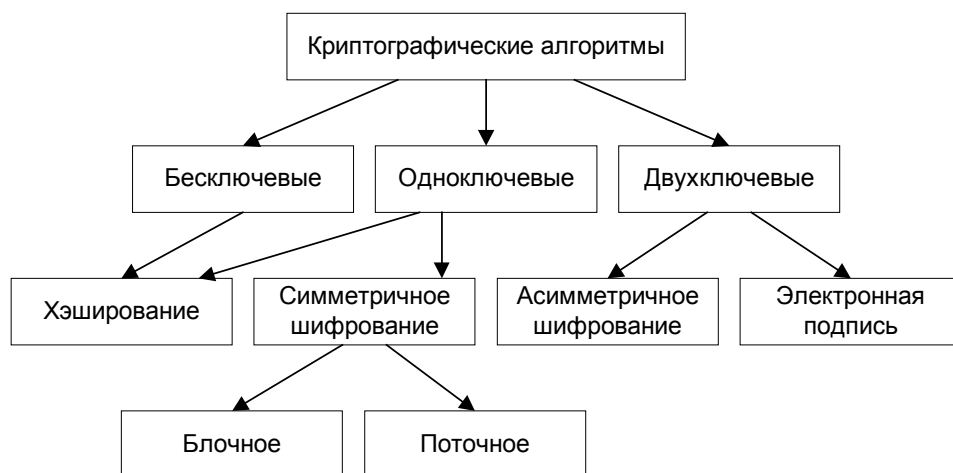
Рис. 4.2. Классификация криптоалгоритмов защиты информации
