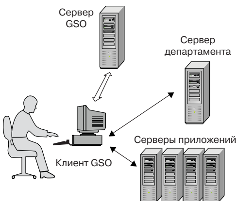
Рис. 5.12. Базовые компоненты GSO
