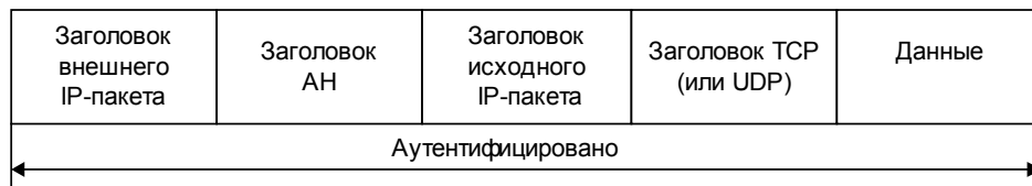
Рис. 8.13. IP-пакет после применения протокола АН в транспортном и туннельном режимах
