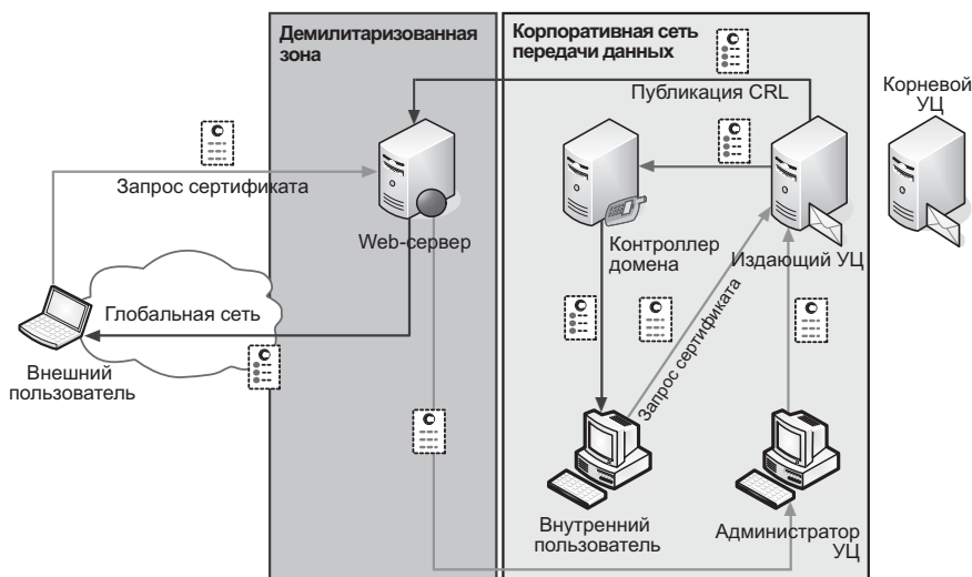
Рис. 4.30. Схема инфраструктуры открытых ключей на базе продуктов Microsoft Active Directory и Microsoft Certification Authority
