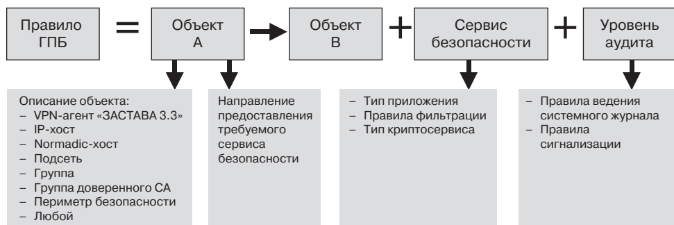
Рис. 14.2. Структура правила глобальной политики безопасности
