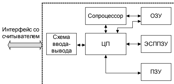
Рис. 5.3. Блок-схема микроконтроллера, встраиваемого в микропроцессорную смарт-карту
