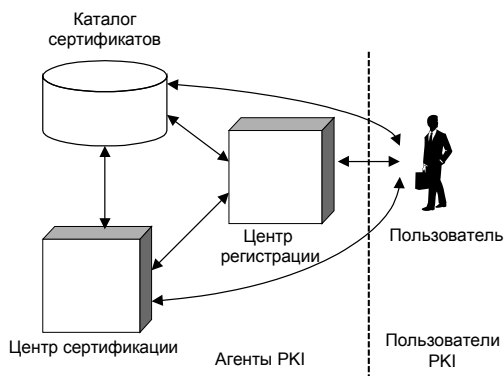
Рис. 4.29. Структура PKI
