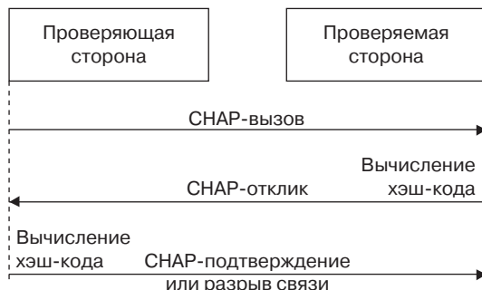
Рис. 11.6. Шаги процесса аутентификации по протоколу CHAP
