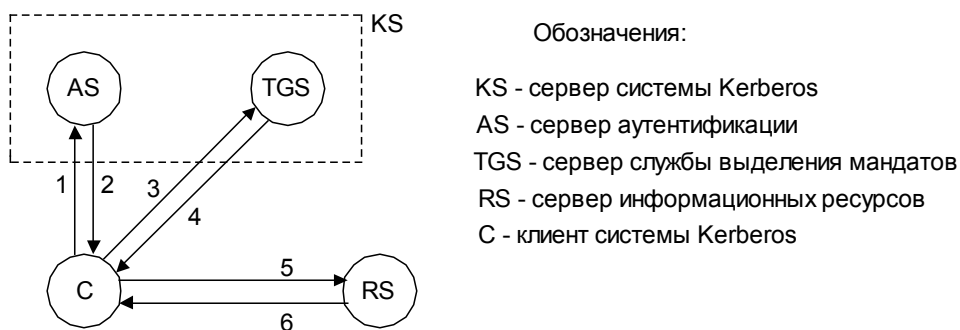
Рис. 11.8. Схема работы протокола Kerberos
