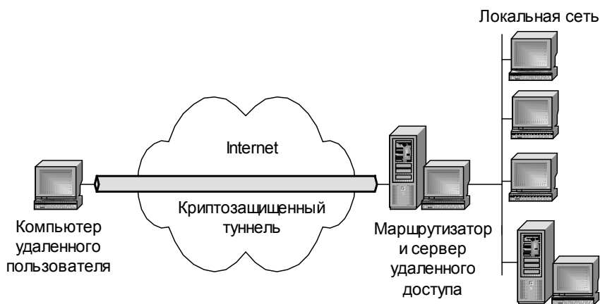
Рис. 8.6. Схема туннелирования при прямом подключении компьютера удаленного пользователя к Интернету
