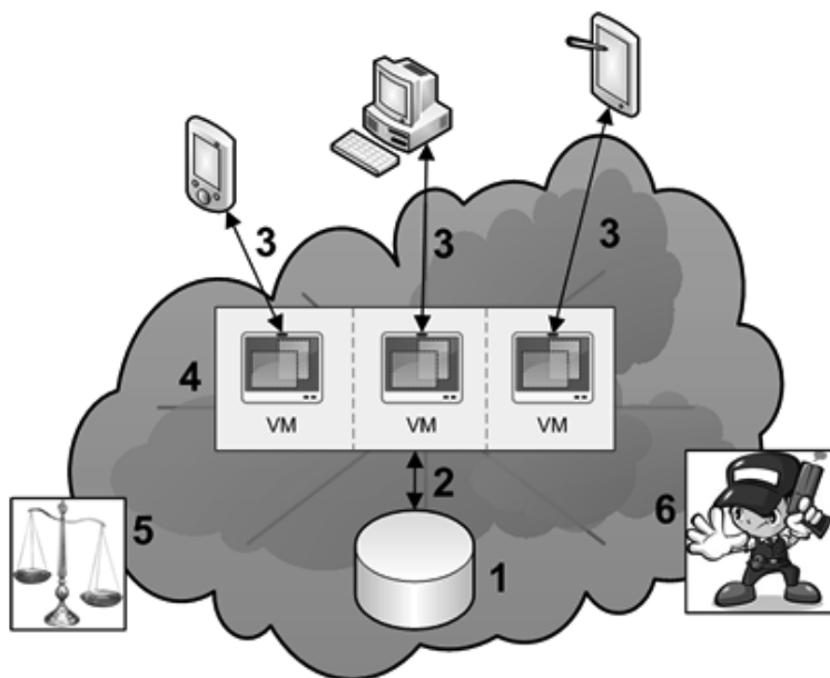
Рис. 6.9. Области безопасности, требующие изучения при выборе провайдера облачных услуг: 1 – защита хранимых данных; 2 – защита данных при передаче; 3 – аутентификация; 4 – изоляция пользователей; 5 – нормативно-правовые вопросы; 6 – реакция на инциденты
