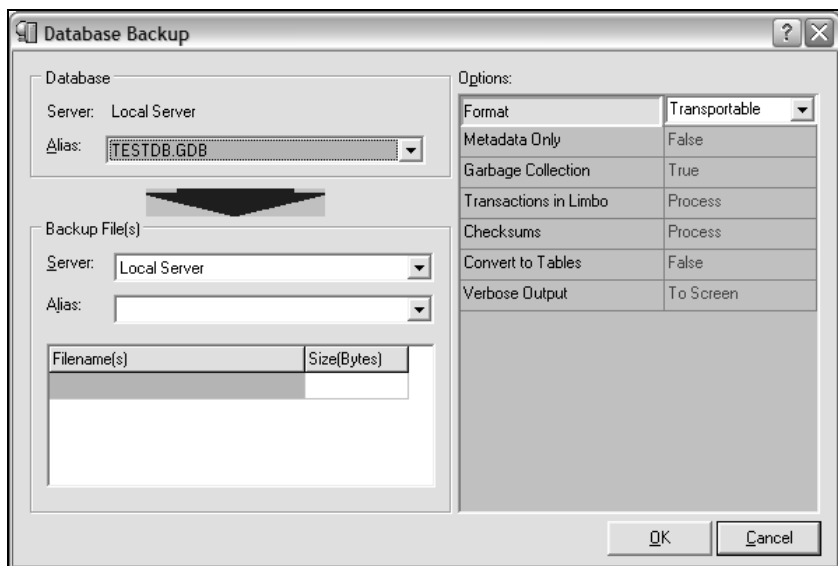
Рис. 7.19. Окно Database Backup
