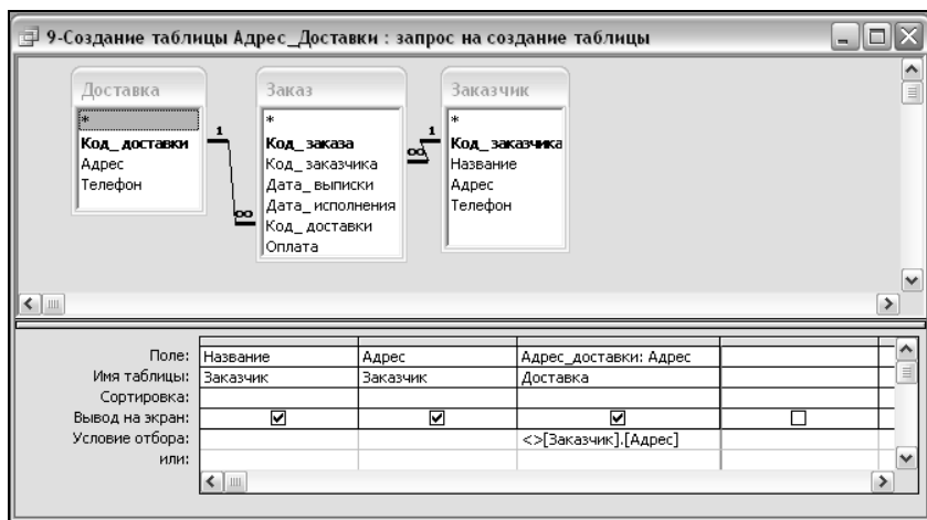
Рис. 6.54. Запрос на создание таблицы
