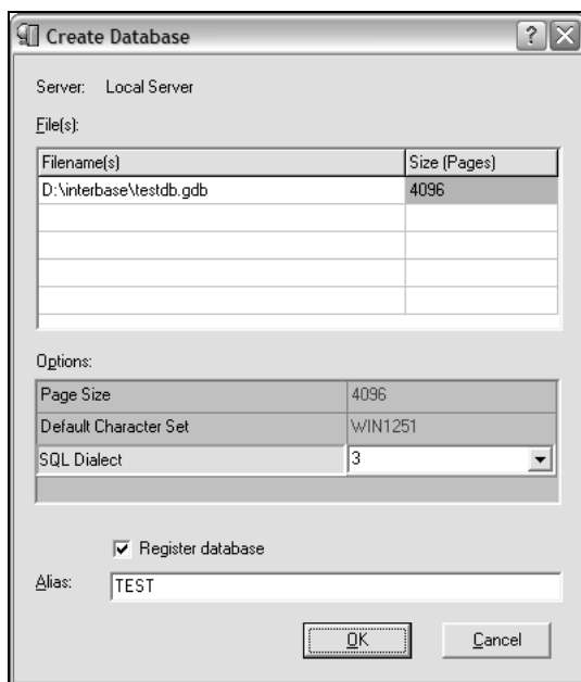
Рис. 7.8. Окно Create Database
