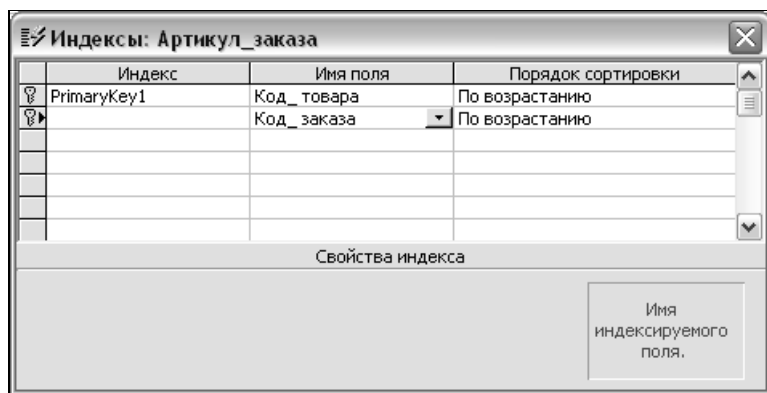
Рис. 6.17. Диалоговое окно Индексы
