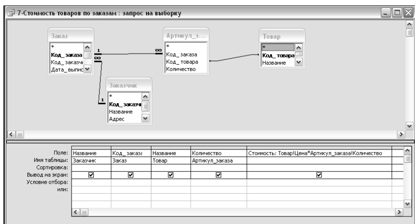
Рис. 6.51. Запрос с вычисляемым полем
