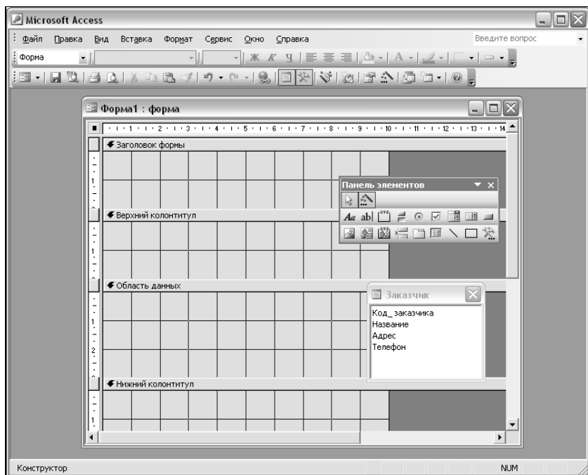
Рис. 6.70. Окно конструктора формы
