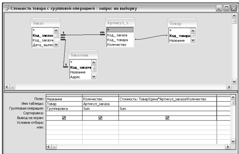
Рис. 6.52. Запрос с вычисляемым полем и групповой операцией
