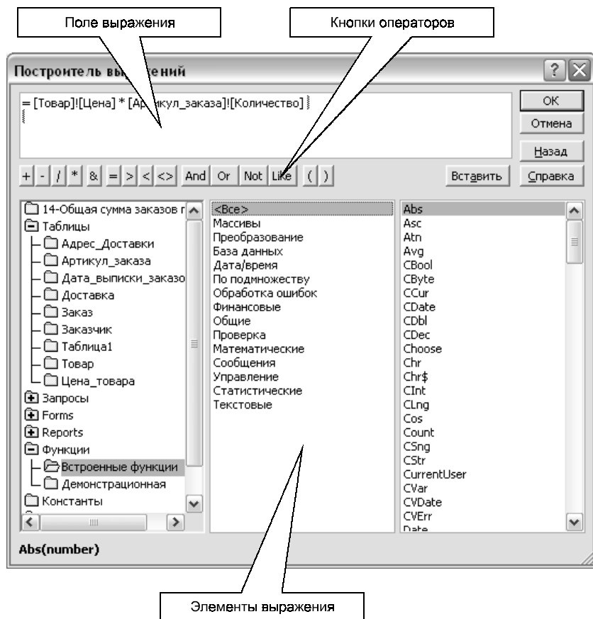
Рис. 6.23. Окно Построитель выражений
