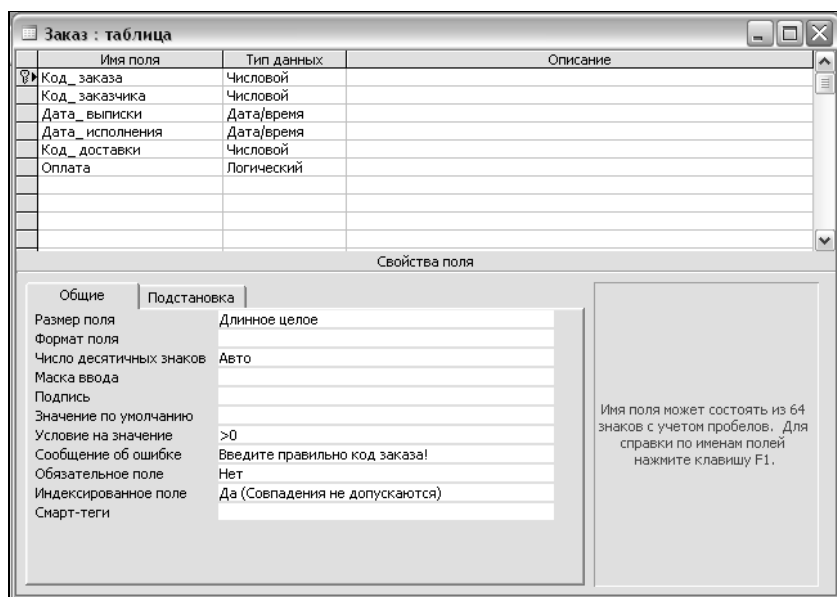
Рис. 6.13. Окно конструктора таблиц
