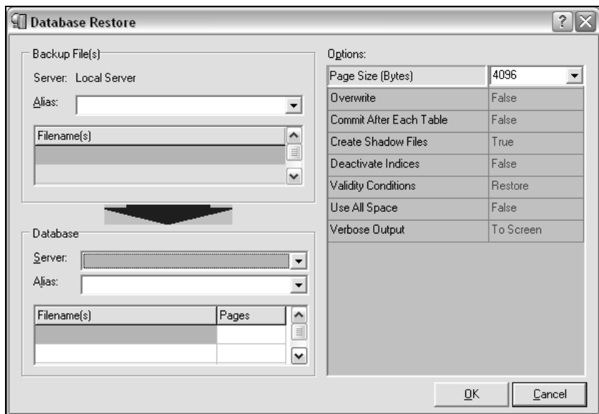
Рис. 7.20. Установка параметров для восстановления базы данных в окне Database Restore
