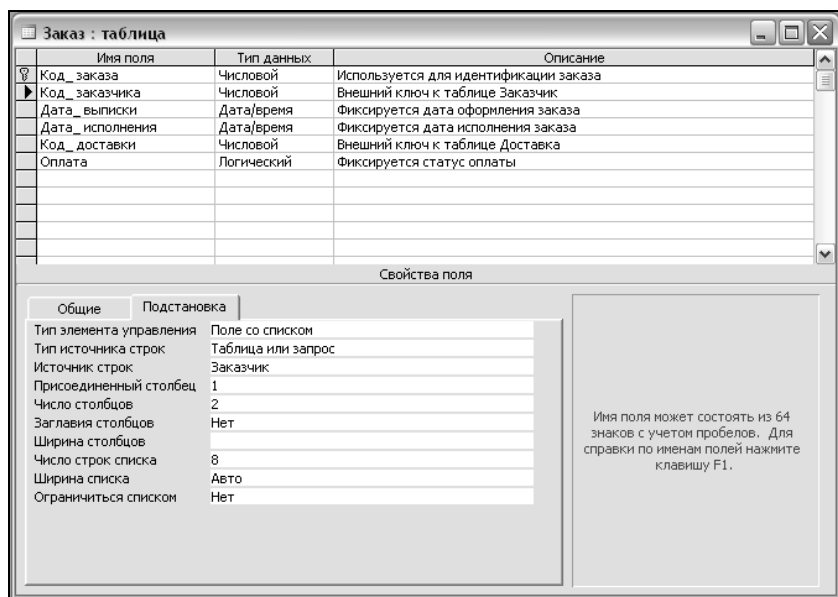
Рис. 6.30. Установка свойств поля на вкладке Подстановка для поля Код_заказчика табл. 6.10
