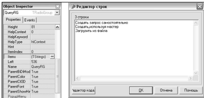
Рис. 7.46. Изменение свойства Items компонента QueryRG ( RadioGroup )
