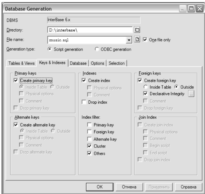
Рис. 7.30. Окно Database Generation — вкладка Keys & Indexes
