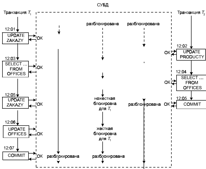
Рис. 5.4. Жесткая и нежесткая блокировки
