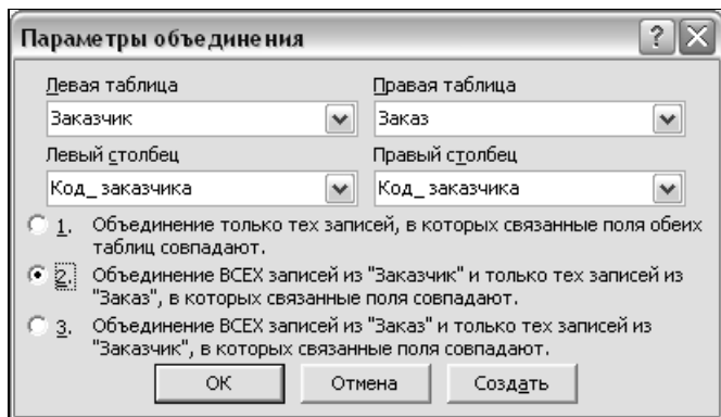
Рис. 6.47. Диалоговое окно Параметры объединения при изменении связи в запросе
