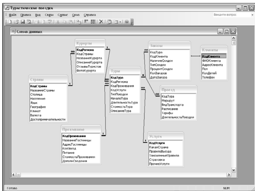
Рис. 6.5. Окно Схема данных
