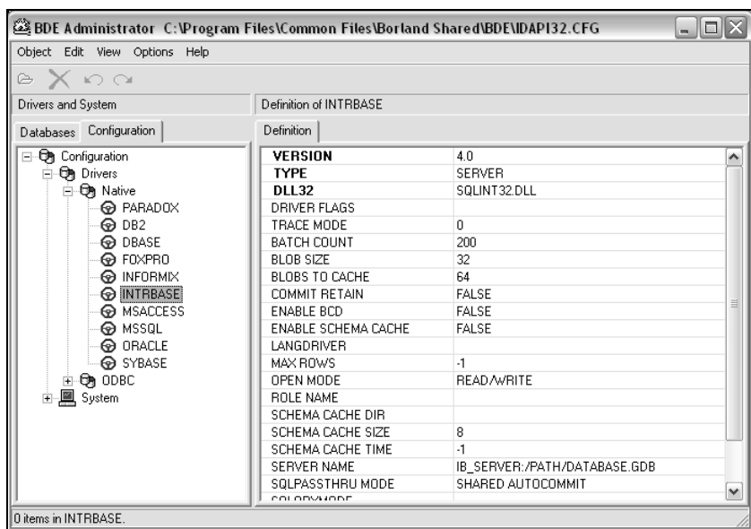
Рис. 7.24. Установка необходимых параметров драйвера
