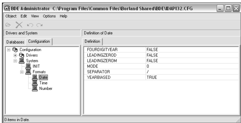
Рис. 7.26. Окно BDE Administrator для изменения форматов даты, времени и числовых значений
