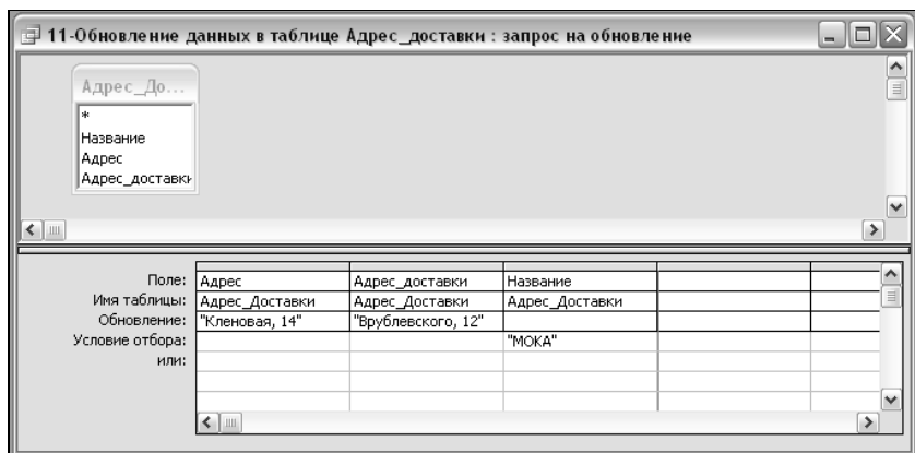
Рис. 6.57. Запрос на обновление
