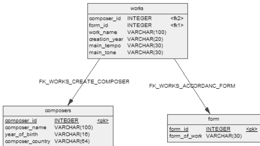
Рис. 7.28. Физическая модель для базы данных "Музыкальные произведения"
