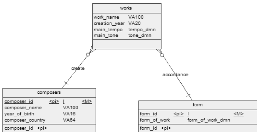
Рис. 7.27. Концептуальная диаграмма для базы данных "Музыкальные произведения"
