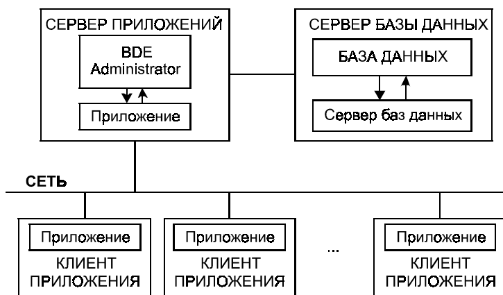
Рис. 7.3. Трехзвенная архитектура "клиент-сервер"
