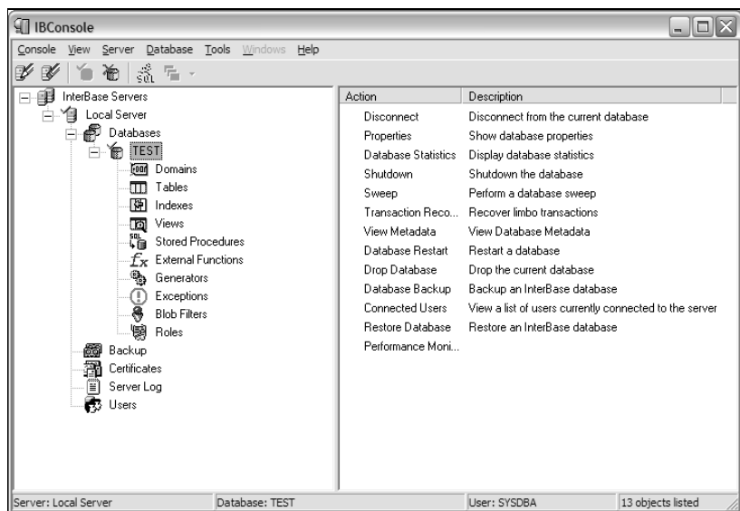
Рис. 7.9. Объекты базы данных в окне IBConsole
