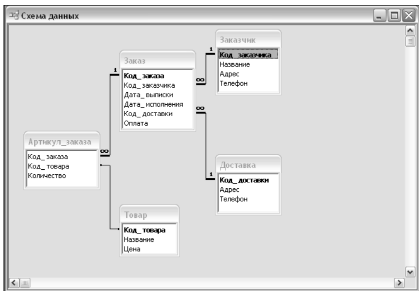
Рис. 6.19. Окно Схема данных
