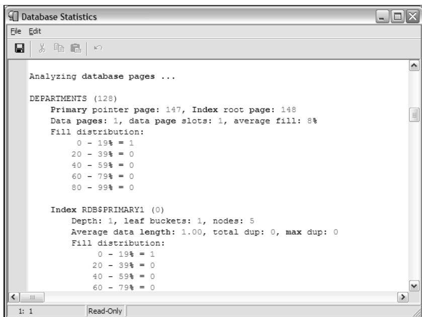
Рис. 7.17. Информация о таблицах базы данных в окне Database Statistics
