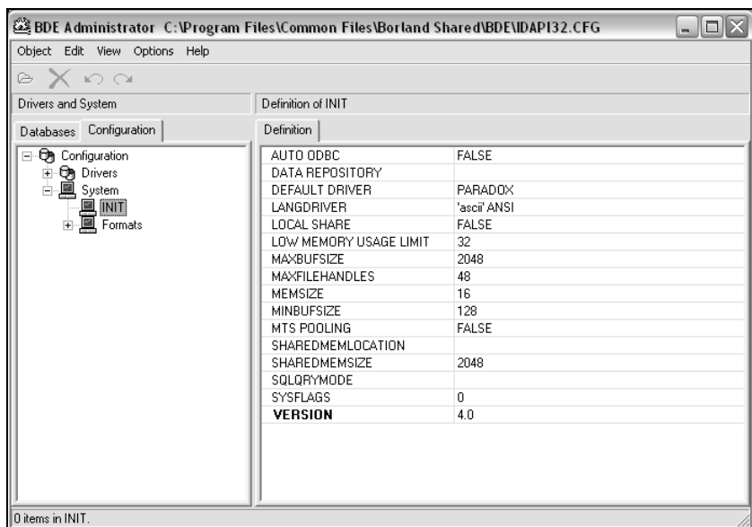
Рис. 7.25. Окно BDE Administrator для изменения системных установок
