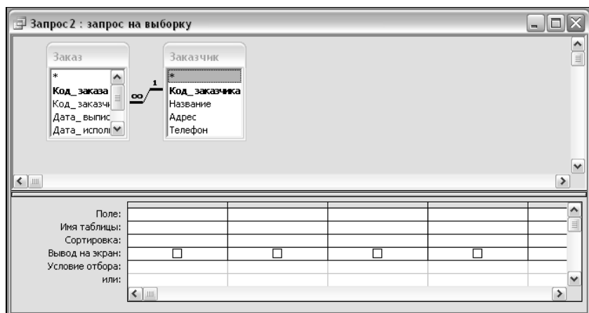
Рис. 6.35. Окно конструктора запроса с таблицами "Заказ" и "Заказчик"
