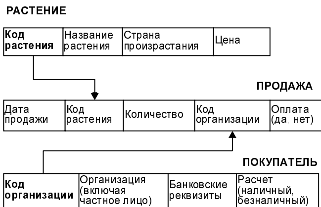
Рис. 3.2. Схема базы данных "Цветочный магазин"
