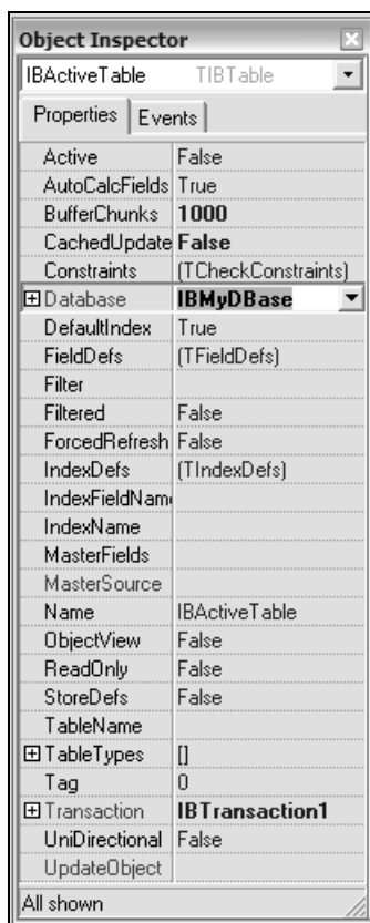
Рис. 7.44. Установка свойств для компонента IBTable
