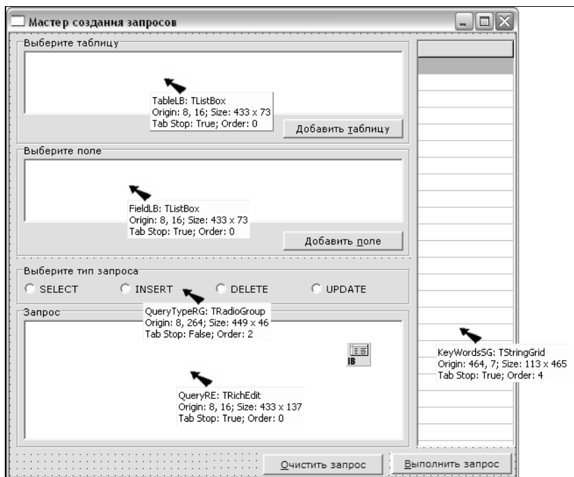
Рис. 7.56. Форма для построения мастера запросов на стадии разработки
