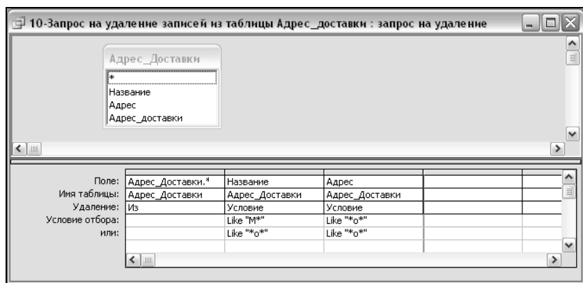
Рис. 6.56. Запрос на удаление
