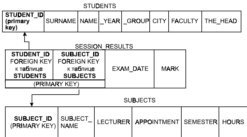
Рис. 4.4. Схема базы данных "Студенты" (обобщенная)
