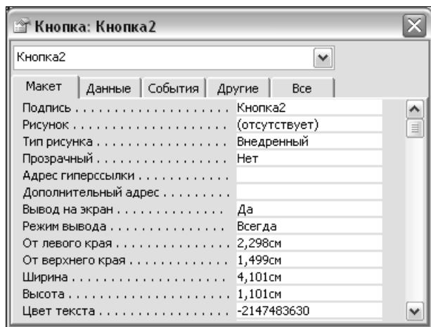
Рис. 6.73. Окно свойств элемента управления
