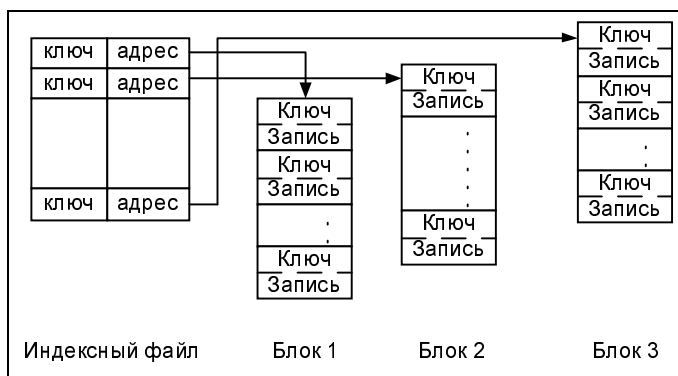
Рис. 2.2. Одноуровневая схема индексации
