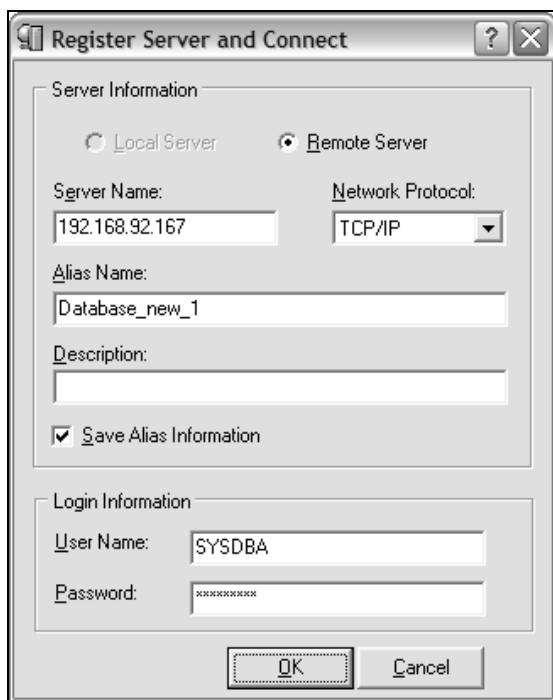
Рис. 7.6. Регистрация удаленного сервера в окне Register Server and Connect
