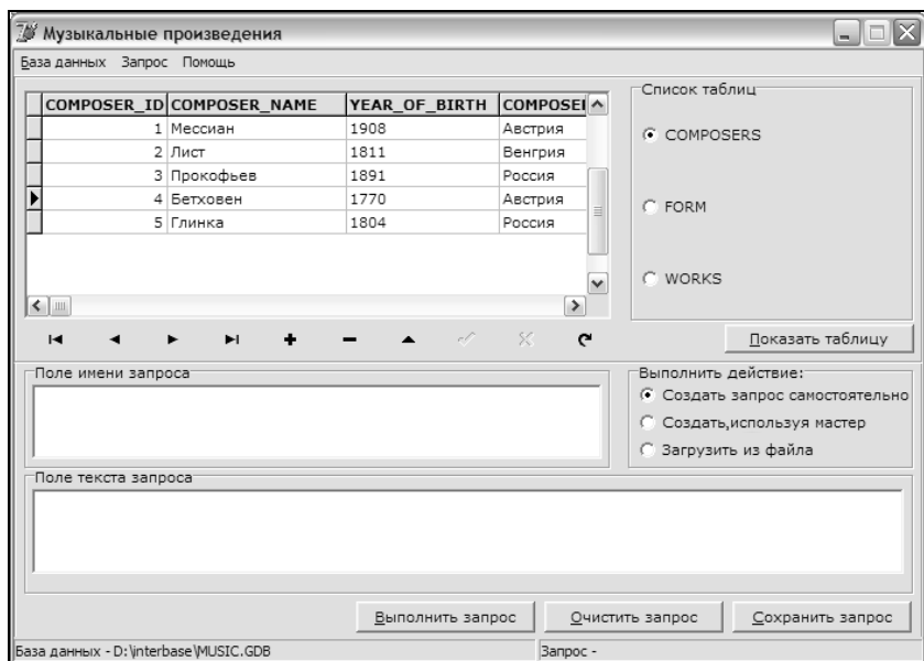
Рис. 7.57. Окно клиентского приложения "Музыкальные произведения"
