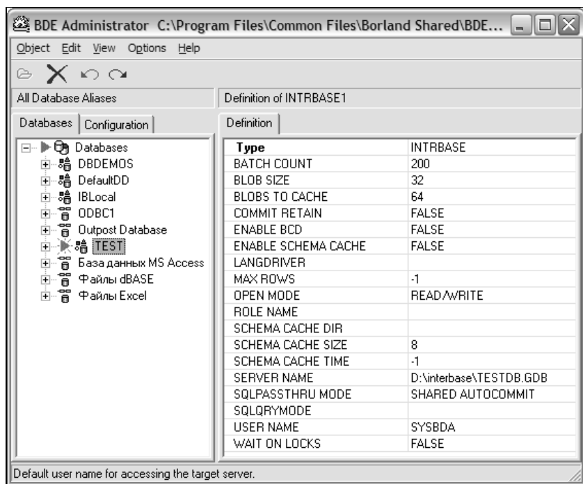
Рис. 7.23. Окно утилиты BDE Administrator
