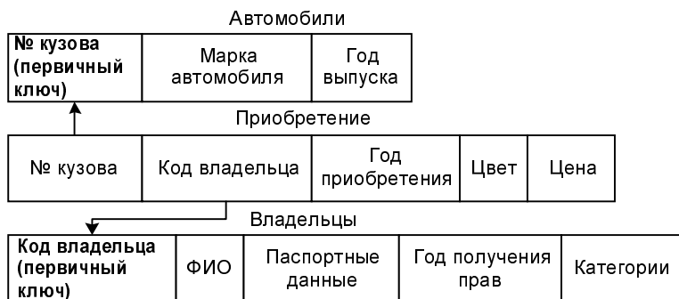
Рис. 7.60. Схема для базы данных "Автомобили"
