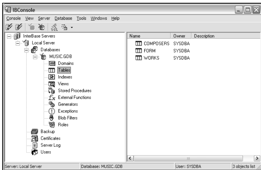
Рис. 7.36. Объекты базы данных "Музыкальные произведения" в окне IBConsole
