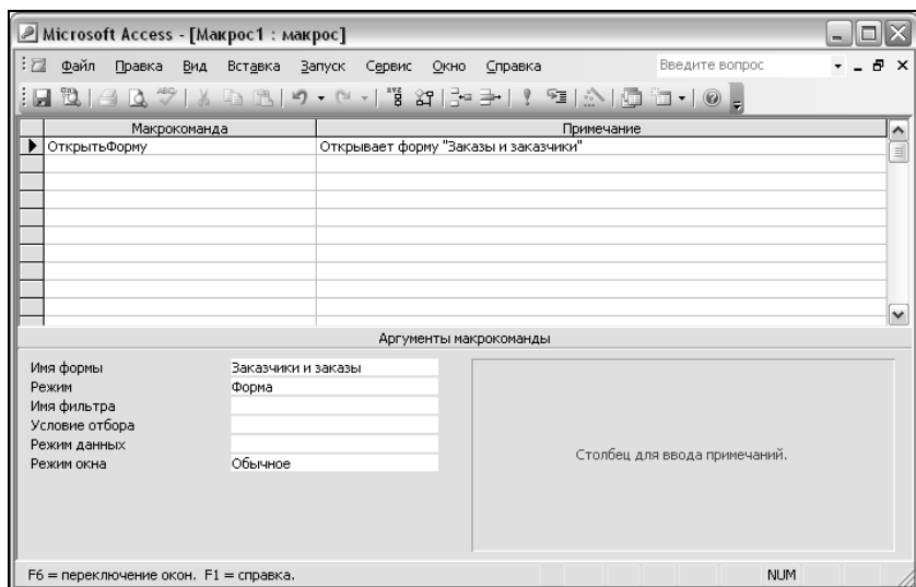
Рис. 6.85. Окно конструктора макросов
