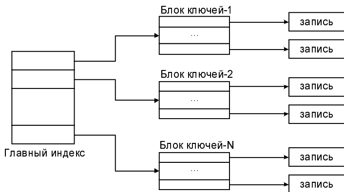
Рис. 2.3. Двухуровневая схема индексации
