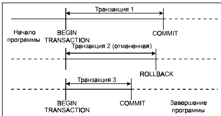
Рис. 5.1. Программа как согласованность транзакций
