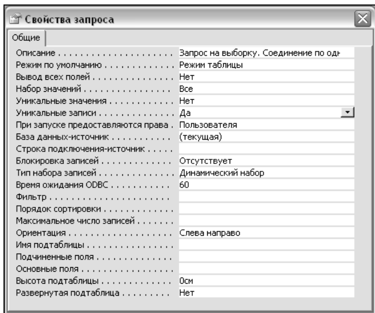
Рис. 6.42. Диалоговое окно Свойства запроса
