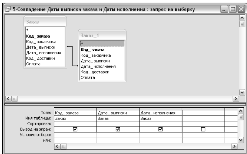
Рис. 6.48. Рекурсивное соединение
