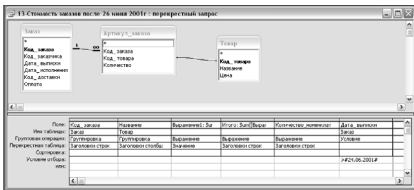
Рис. 6.59. Перекрестный запрос
