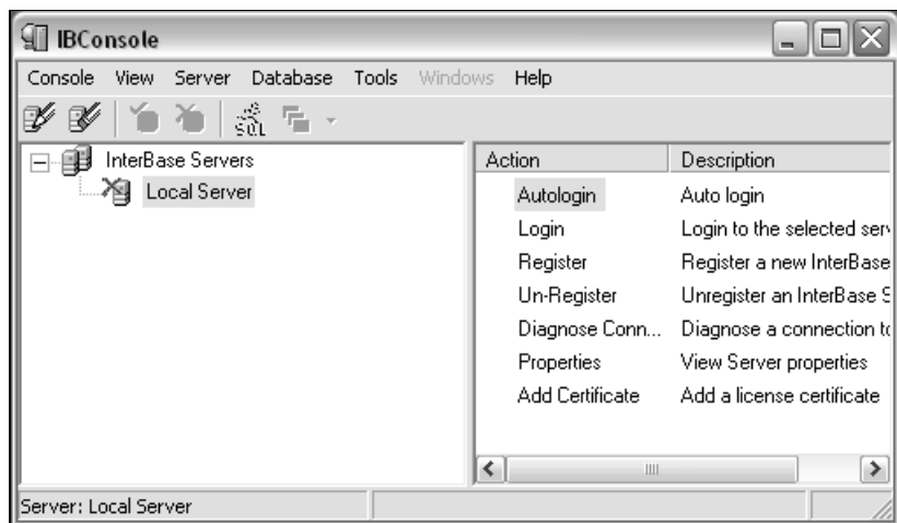
Рис. 7.4. Утилита IBConsole
