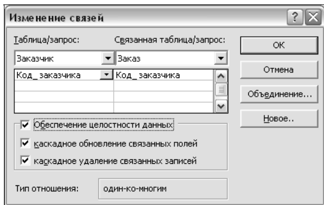
Рис. 6.20. Диалоговое окно Изменение связей
