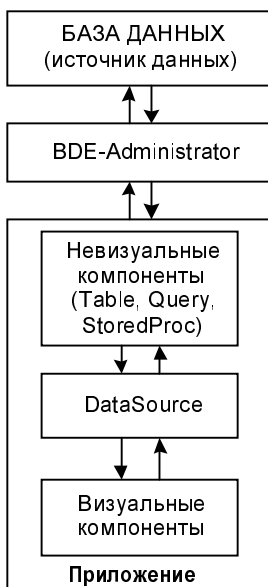
Рис. 7.1. Схема взаимодействия программ с данными
