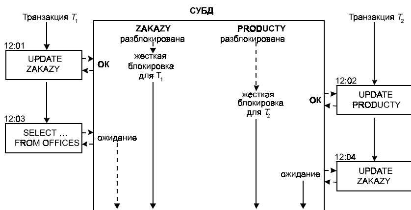
Рис. 5.5. Тупиковая ситуация двух транзакций
