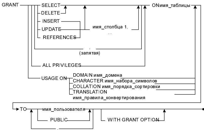
Рис. 5.7. Инструкция предоставления привилегий ( GRANT )
