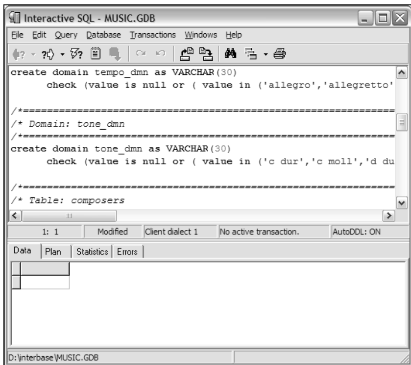
Рис. 7.35. Утилита Interactive SQL с SQL-скриптом для создания базы данных
