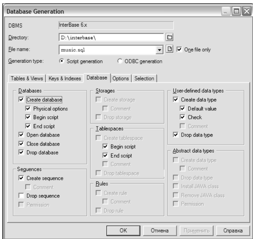
Рис. 7.31. Окно Database Generation — вкладка Database
