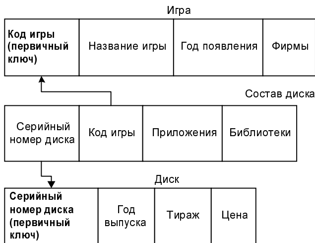
Рис. 7.62. Схема для базы данных "Компьютерные игры"
