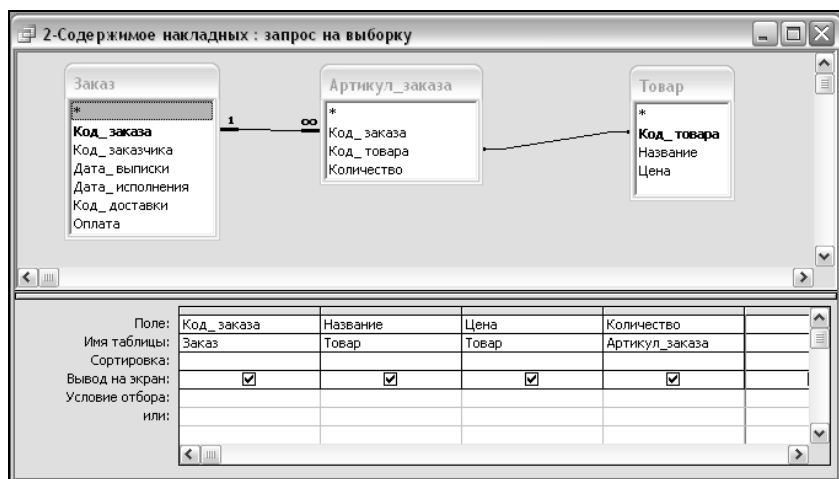
Рис. 6.44. Запрос на выборку с косвенными связями
