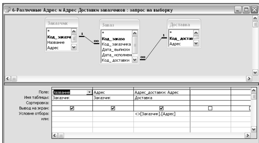
Рис. 6.32. Стандартное окно конструктора запросов
