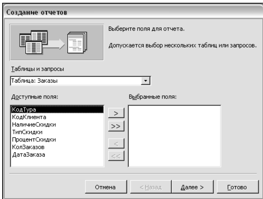
Рис. 6.3. Создание отчета с помощью мастера отчетов
