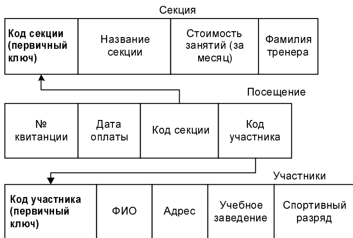
Рис. 7.63. Схема для базы данных "Спортивный клуб"
