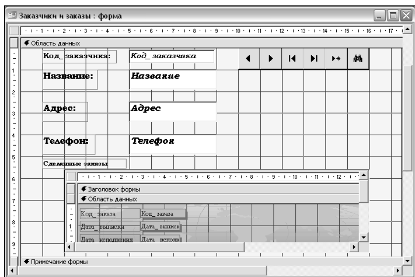
Рис. 6.76. Область данных в режиме конструктор форм
