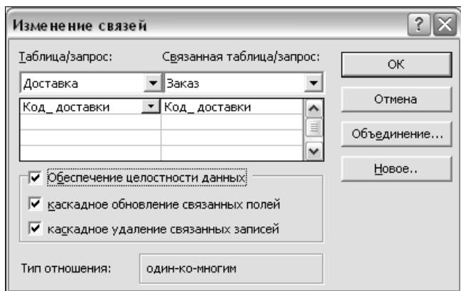
Рис. 6.29. Задание параметров связи в диалоговом окне Изменение связей
