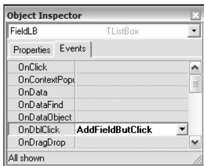
Рис. 7.55. Определение событий для компонента ListBox с именем FieldLB
