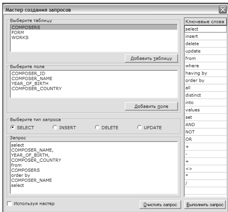
Рис. 7.58. Окно мастера построения запросов клиентского приложения "Музыкальные произведения"
