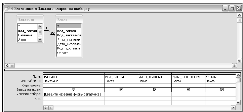
Рис. 6.39. Задание параметра ввода в строке Условие отбора
