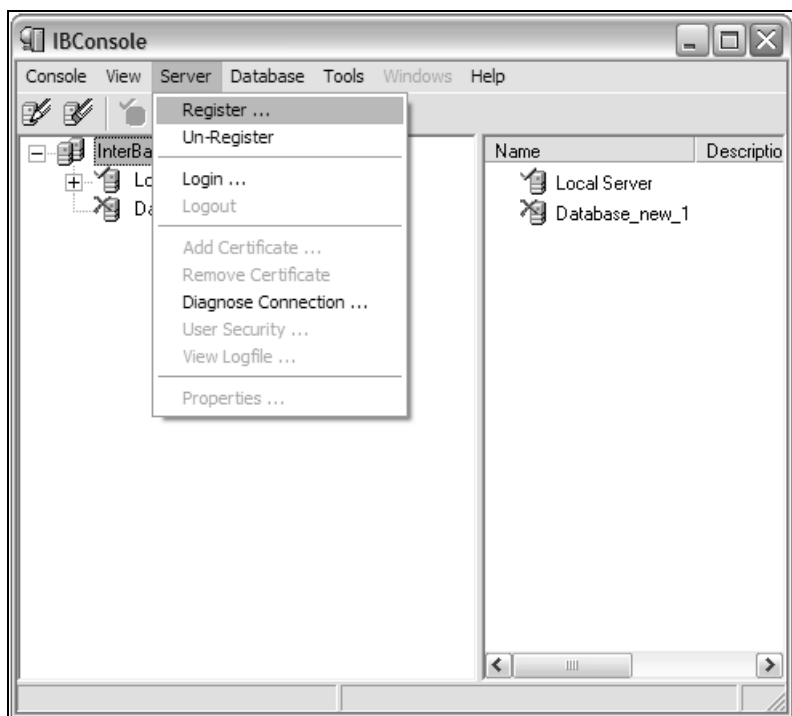
Рис. 7.5. Выбор команды для регистрации локального сервера либо для соединения с удаленным сервером базы данных
