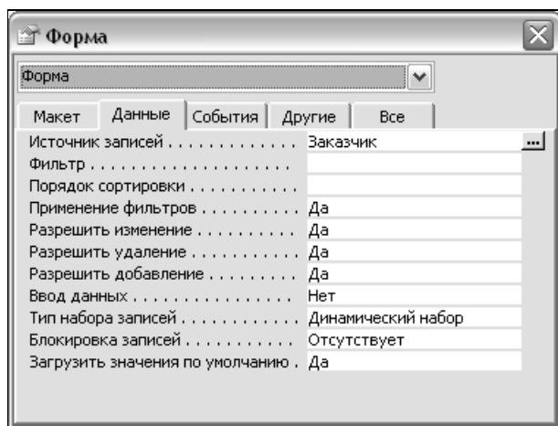
Рис. 6.75. Задание таблицы Заказчик в качестве источника данных для формы
