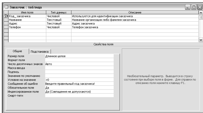
Рис. 6.25. Заполнение диалогового окна конструктора таблиц для создания новой таблицы
