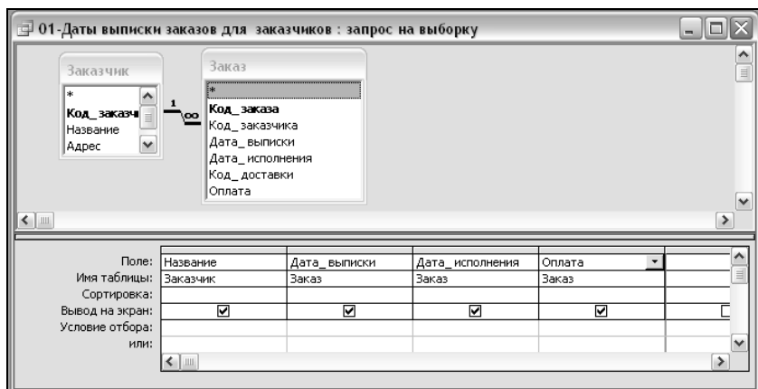
Рис. 6.41. Внутреннее соединение по одному полю
