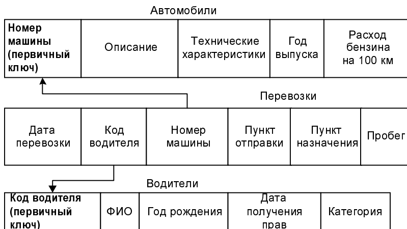
Рис. 7.61. Схема для базы данных "Грузоперевозки"
