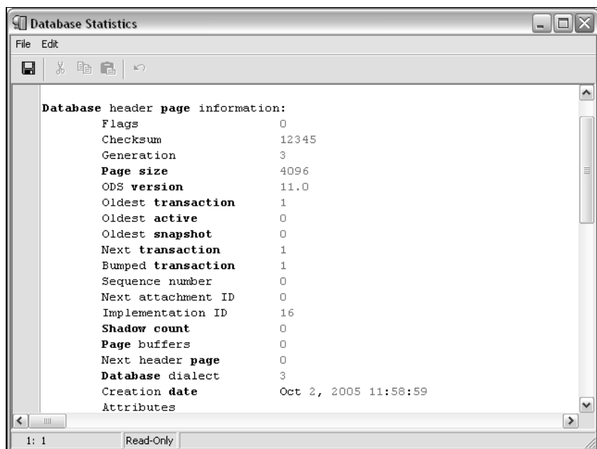
Рис. 7.16. Вывод статистических данных о базе данных в окне Database Statistics
