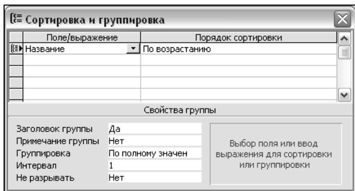
Рис. 6.83. Диалоговое окно Сортировка и группировка
