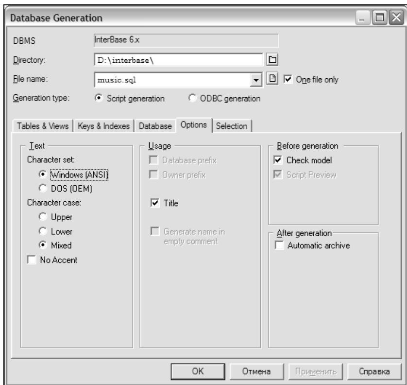
Рис. 7.32. Окно Database Generation — вкладка Options
