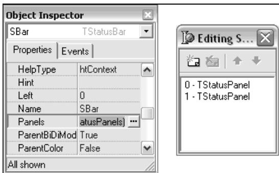
Рис. 7.50. Добавление разделов в свойство Panels компонента StatusBar
