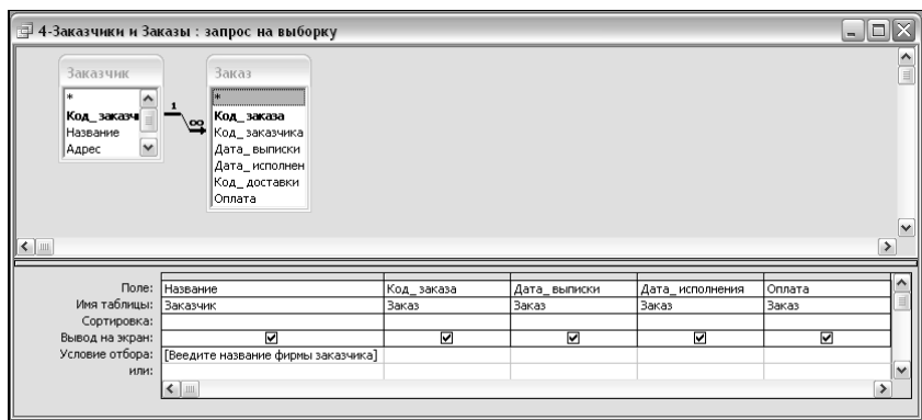
Рис. 6.46. Левое внешнее соединение
