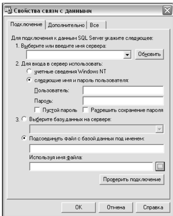
Рис. 6.8. Диалоговое окно Свойства связи с данными
