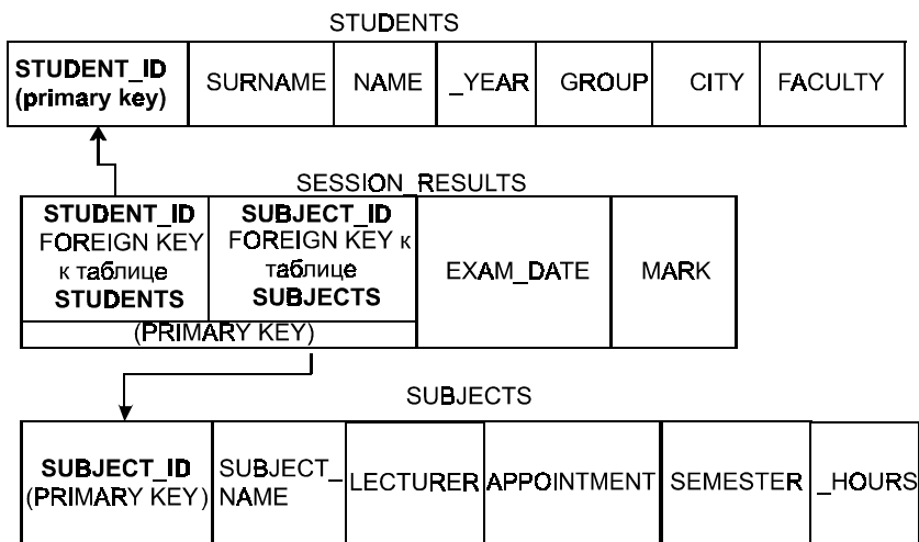
Рис. 4.3. Схема базы данных "Студенты"
