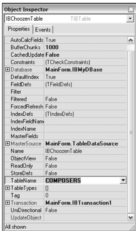
Рис. 7.53. Определение свойств компонента IBTable
