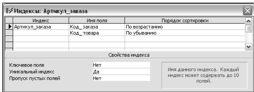
Рис. 6.26. Задание индекса для табл. 6.11
