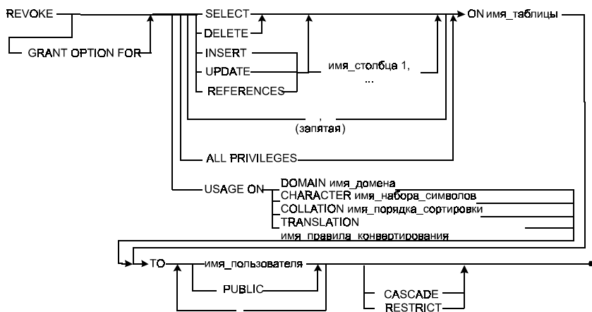
Рис. 5.8. Инструкция отмены привилегий (REVOKE)
