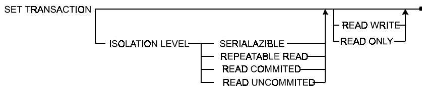
Рис. 5.6. Диаграмма инструкции SET TRANSACTION
