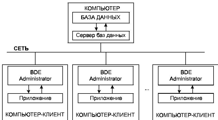
Рис. 7.2. Двухзвенная архитектура "клиент-сервер"
