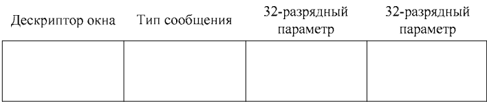
Рис. 1.7. Структура сообщения WM_DESTROY
