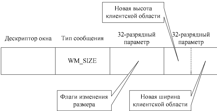
Рис. 1.8. Структура сообщения WM_SIZE
