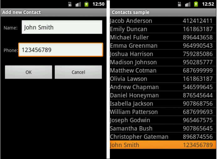
Рис. 12.10. Вставка новой записи из окна дочернего Activity
