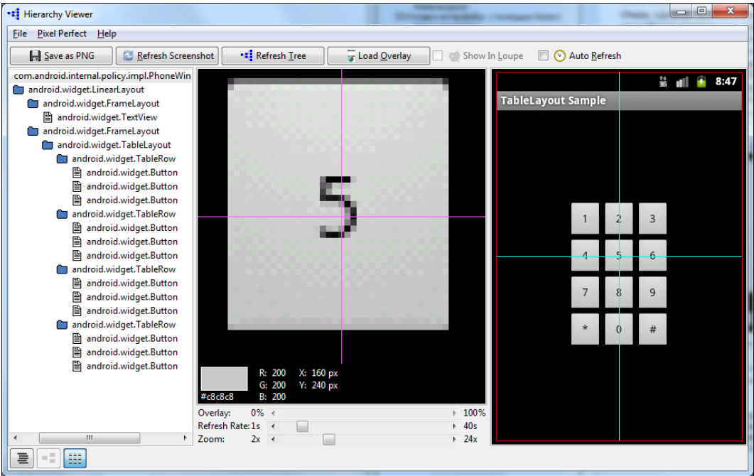
Рис. 4.14. Окно Pixel Perfect View утилиты Hierarchy Viewer
