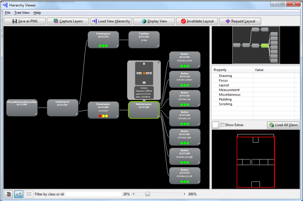
Рис. 4.13. Окно Layout View утилиты Hierarchy Viewer
