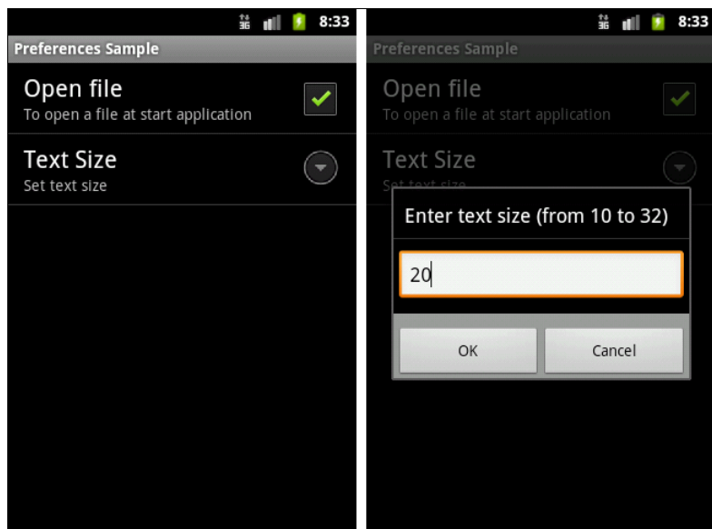
Рис. 16.6. Вызов окна EditTextPreference для установки размера текста
