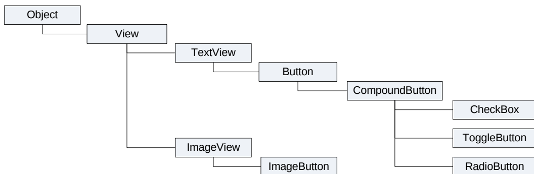
Рис. 6.1. Иерархия классов Button , CheckBox , ToggleButton , RadioButton и ImageButton
