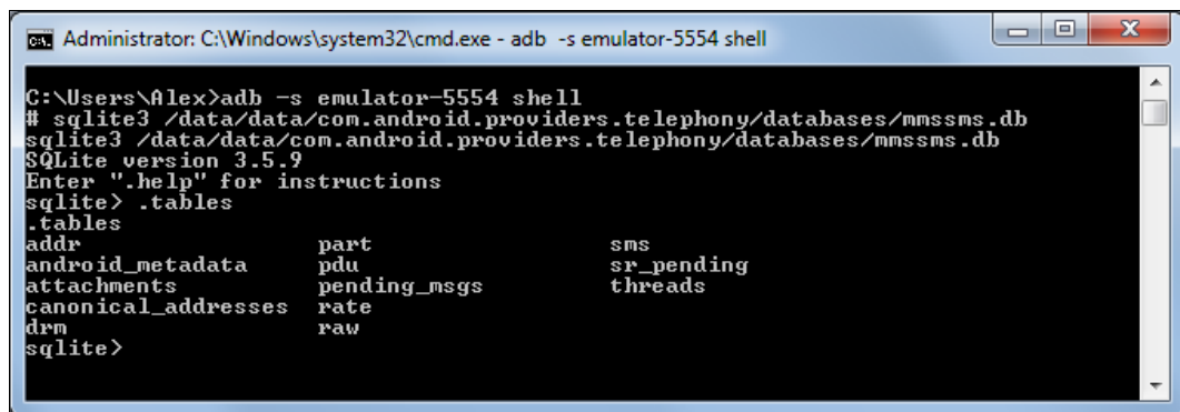
Рис. 15.2. Вывод списка таблиц базы данных SMS- и MMS-сообщений
