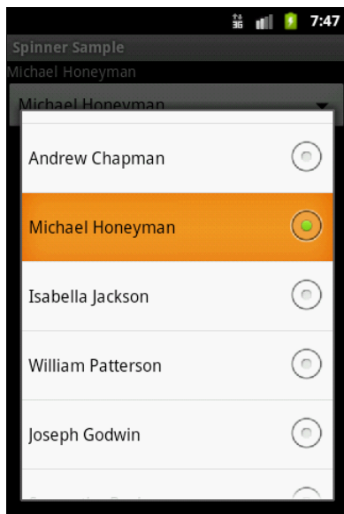
Рис. 8.8. Приложение с виджетом Spinner
