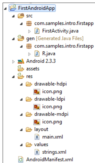
Рис. 3.7. Структура проекта "FirstAndroidApp" в окне Package Explorer
