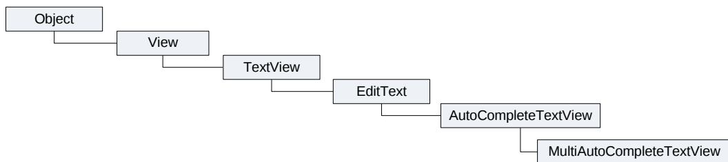
Рис. 8.1. Иерархия классов текстовых полей с автозаполнением
