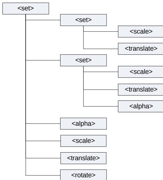
Рис. 19.2. Пример структуры XML-файла анимации
