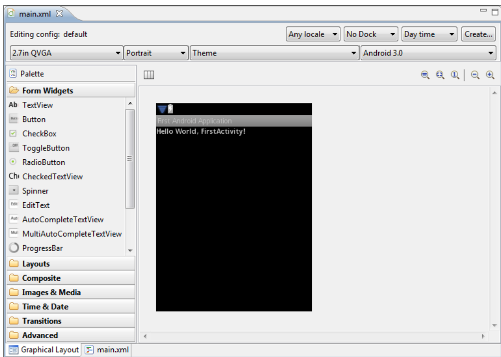
Рис. 3.8. Редактор компоновки
