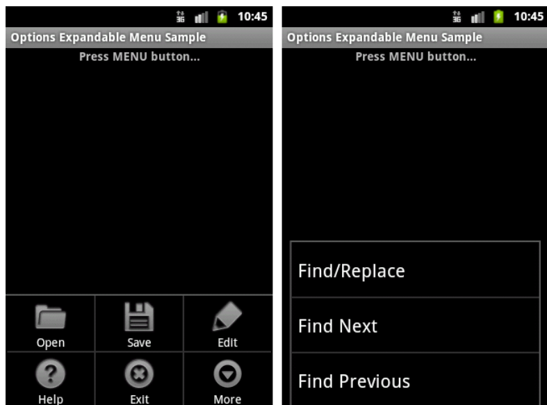
Рис. 11.3. Расширенное меню
