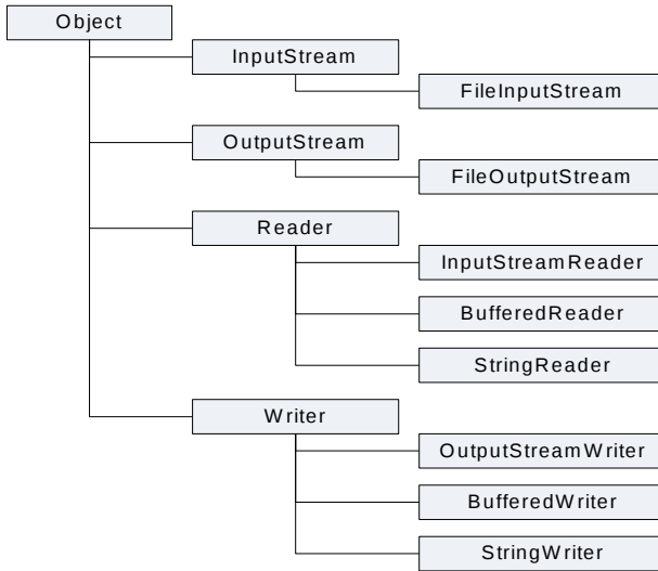
Рис. 16.1. Классы для файлового ввода-вывода в Android
