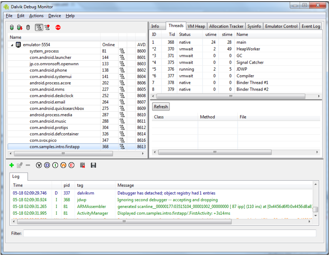
Рис. 3.13. Информация о выполняемом процессе в DDMS
