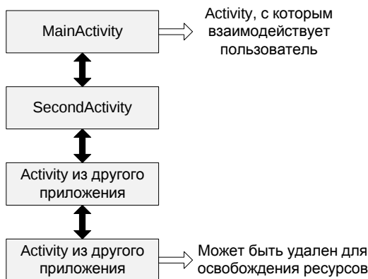
Рис. 12.6. Стек Activity
