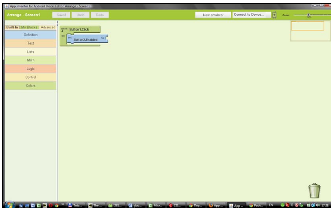
Рис. 12.11. Редактор блоков
