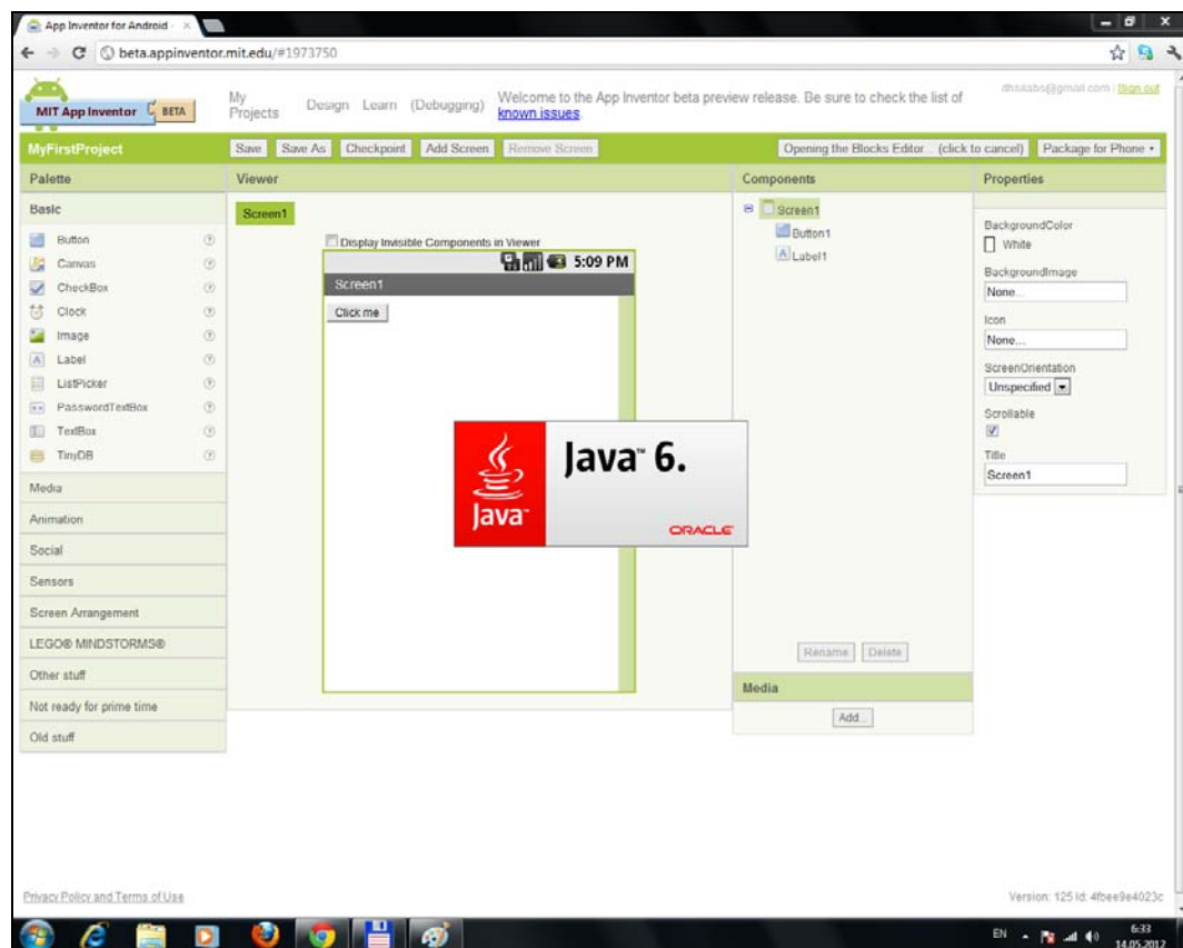
Рис. 10.8. Запуск Java
