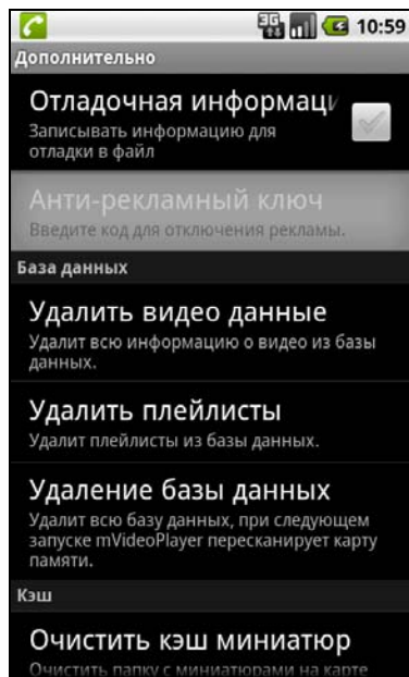
Рис. 2.21. Раздел Дополнительно
