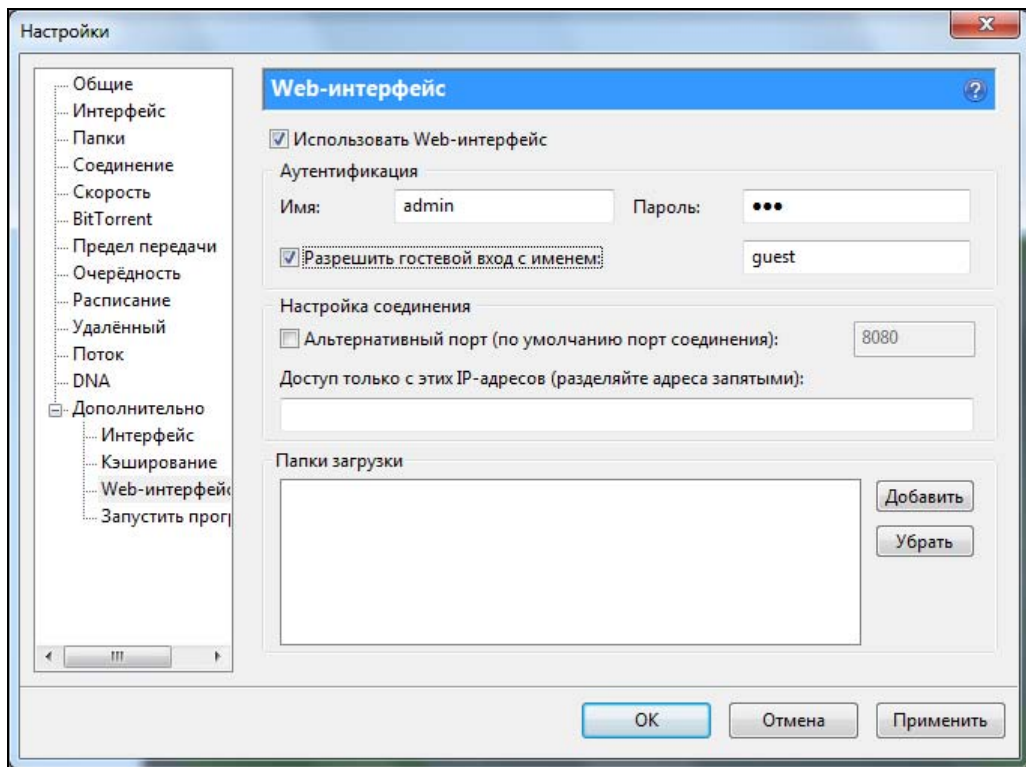
Рис. 3.9. Настройка uTorrent
