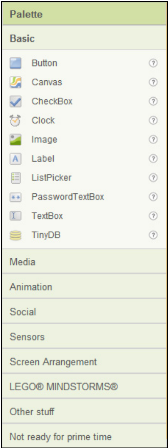
Рис. 12.2. Палитра компонентов
