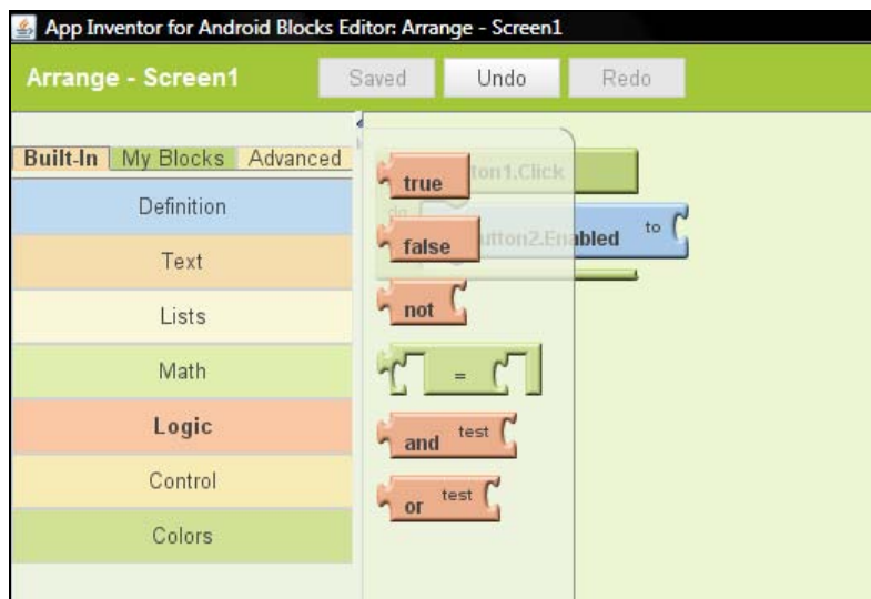
Рис. 12.10. Выбор константы
