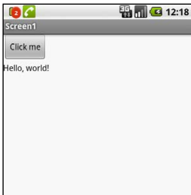
Рис. 11.17. Приложение запущено
