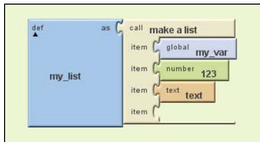
Рис. 12.18. Объявление списка
