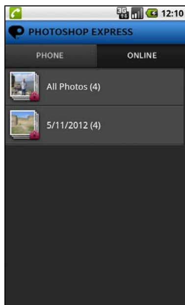
Рис. 2.29. Созданные альбомы
