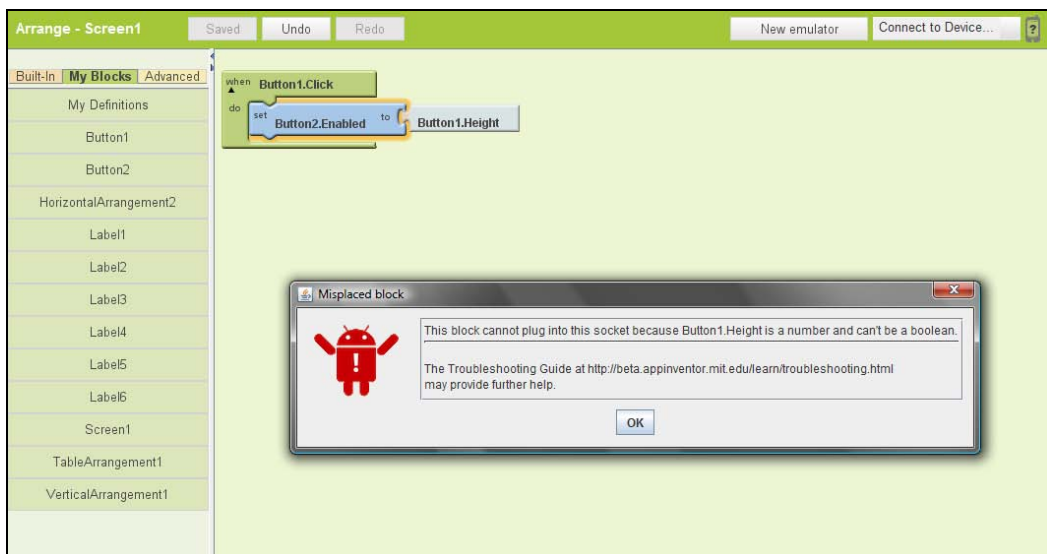
Рис. 12.9. Несовместимость блоков
