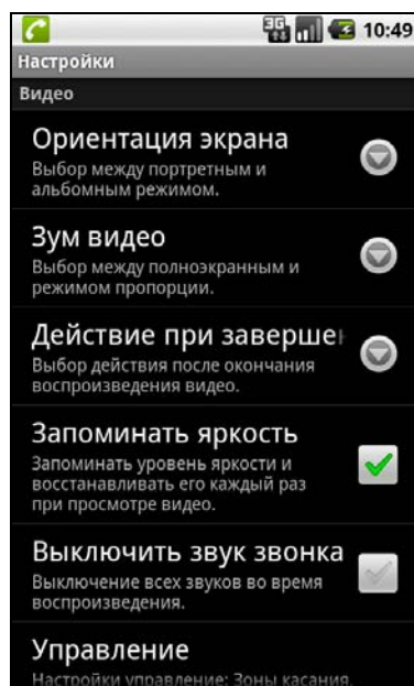
Рис. 2.19. Опции программы
