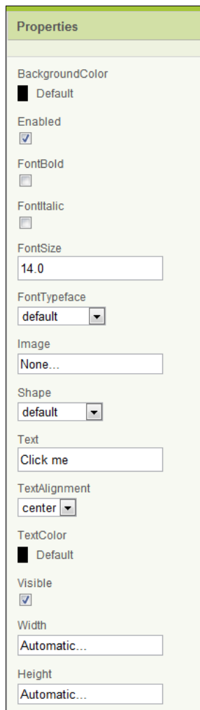
Рис. 11.5. Свойства компонента
