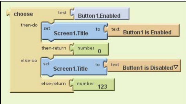
Рис. 12.22. Блок choose
