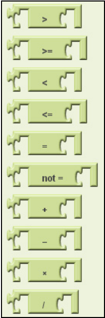
Рис. 12.29. Математические операции
