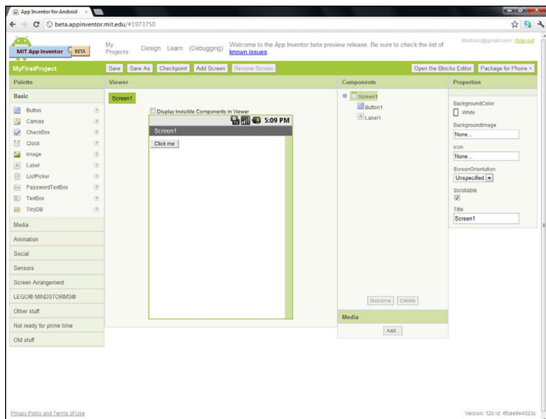
Рис. 10.5. Визуальное проектирование
