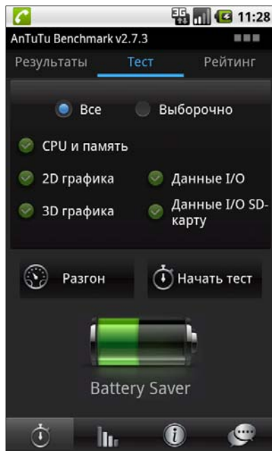
Рис. 8.8. Параметры теста
