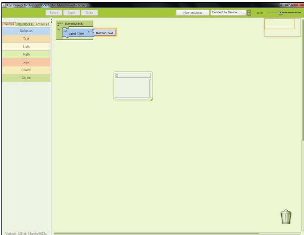
Рис. 10.18. Редактор блоков
