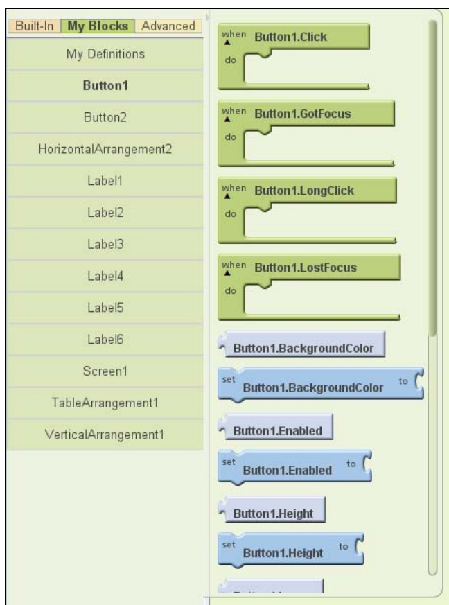
Рис. 12.8. Блоки
