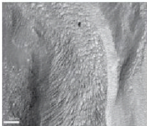
Рис. 12.6 Фотография, сделанная с Mars Reconnaissance Orbiter NASA. Показаны особенности ледохода в древнем русле реки на южной стене кратера Грега. (А). Холмы в нижней части фото изрезаны сухими руслами рек, текущими вниз на север (на фото вверх). Более легкие по текстуре материалы переносились по руслу и скопились на дне кратера (сверху)
