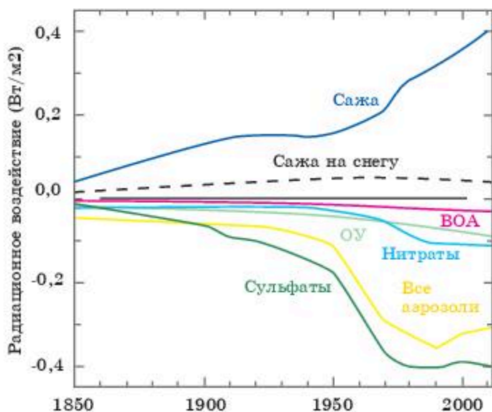
Рис. 12.2. Твердые аэрозольные частицы и сажа
