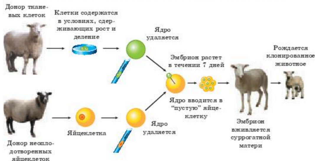
Рис. 9.11. Клонирование животных
