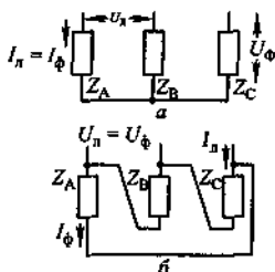
Рис. 1.5. Схемы соединения электроприемников: а — в звезду; б — в треугольник
