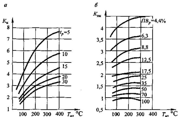
Рис. 10.1. Зависимости расчетных коэффициентов от постоянной времени нагрева для кратковременного ( a ) и повторно-кратковременного ( б ) режимов работы
