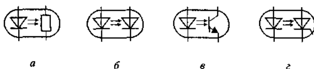
Рис. 11.7. Условные изображения оптопар: а — резисторная; б — диодная; в — транзисторная; г — тиристорная
