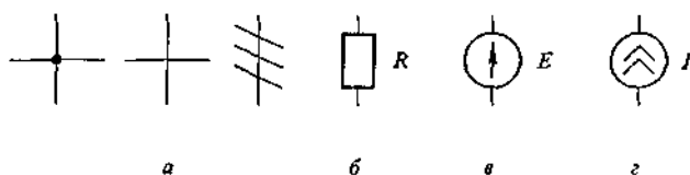
Рис. 1.1. Условные изображения: a – электрических линий; б – активного резистора; в – источника ЭДС; г – источника тока
