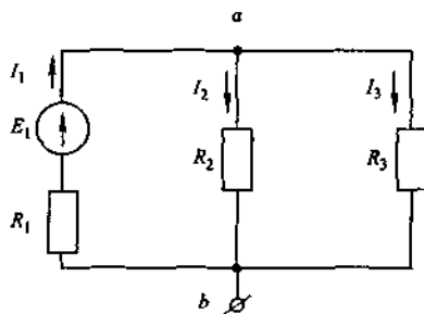
Рис. 1.2. Пример электрической схемы
