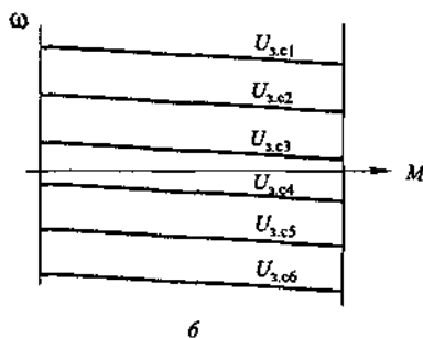
Рис. 13.6. Схема (а) и механические характеристики (б) электропривода с подчиненным регулированием координат
