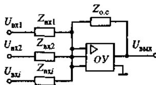
Рис. 11.1. Схема операционного усилителя
