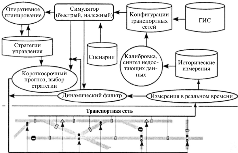
Рис. 4.49. Схема работы АУТС
