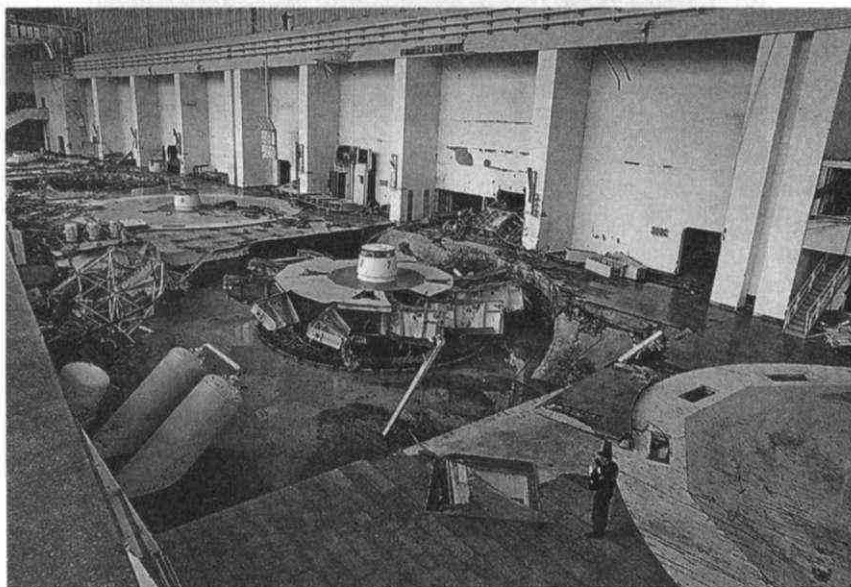
Рис. 19. Авария на Саяно-Шушенской ГЭС
