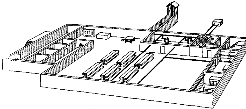
Рис. 35. План встроенного убежища
