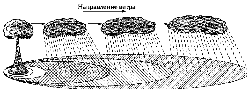
Рис. 29. Образование радиоактивного следа
