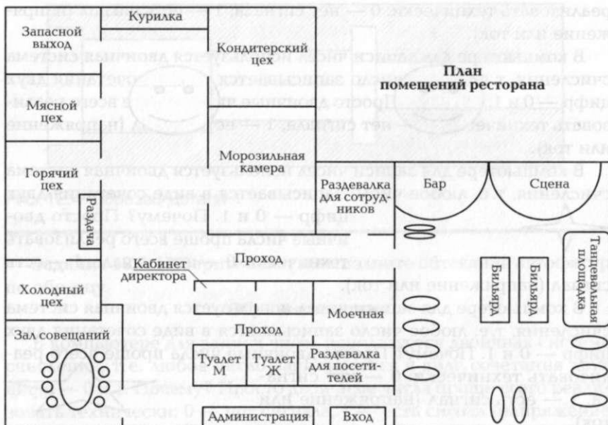
Рис. 12.6. План ресторана
