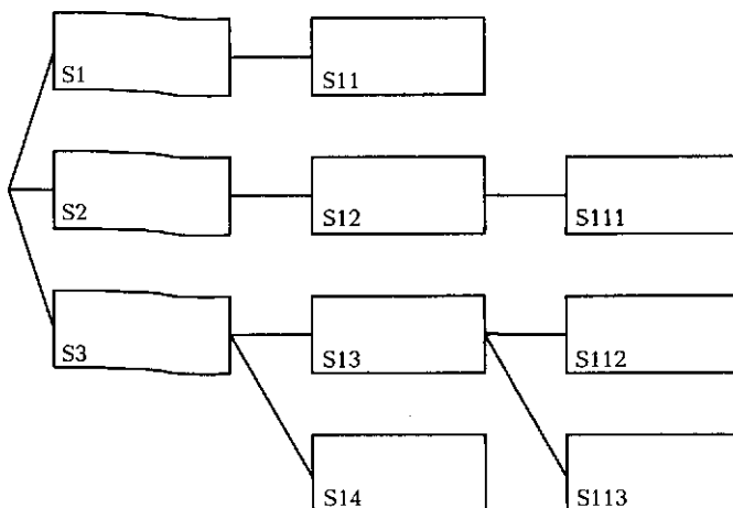
Рис. 7.1. Дерево каталогов
