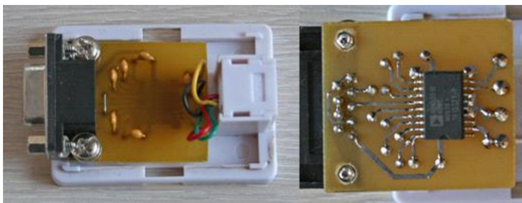
Рис. 58 Адаптер Vaillant с гальванической развязкой на ADM3251
