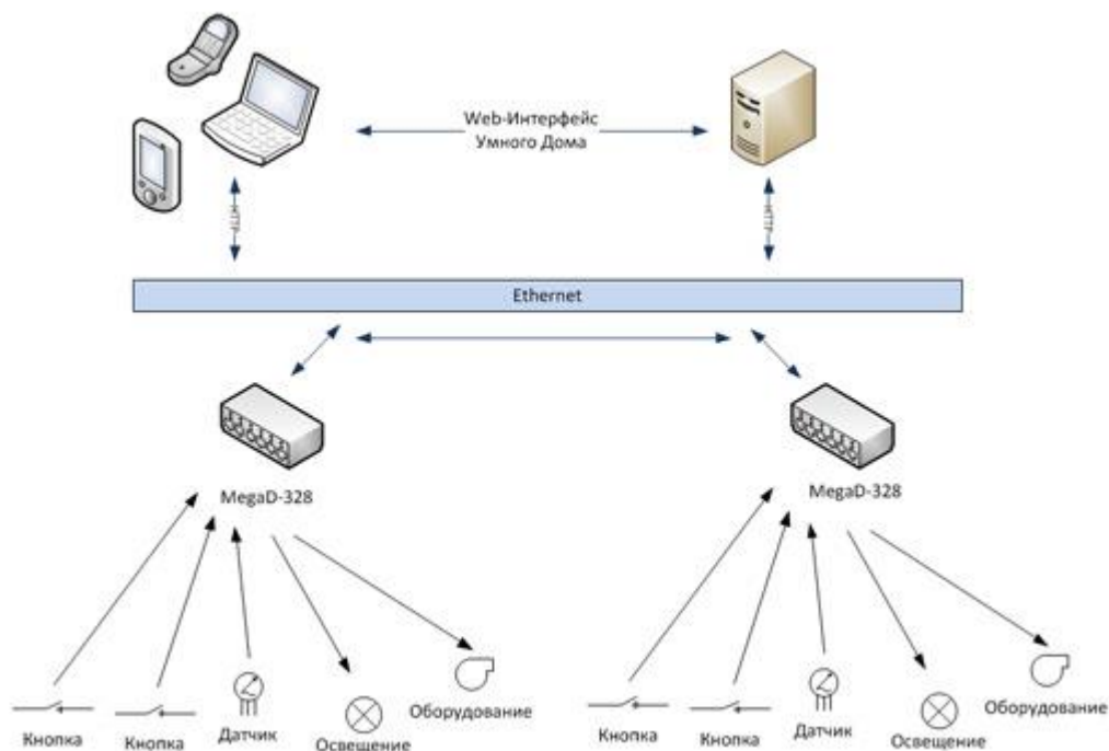
Рис. 36 Схема использования MegaD-328 с сервером. Управление нагрузками как напрямую, так и по команде с сервера.
