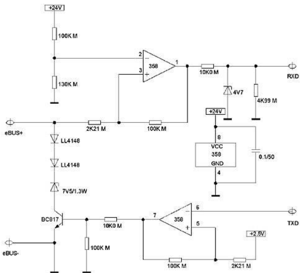
Рис. 64 Принципиальная схема простейшего адаптера E-Bus без гальванической развязки
