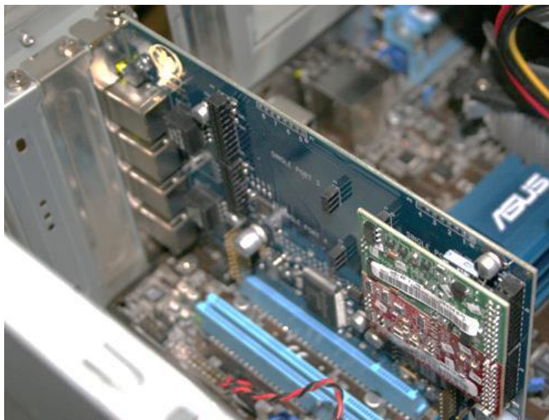
Рис. 90 Плата Digium TDM410
