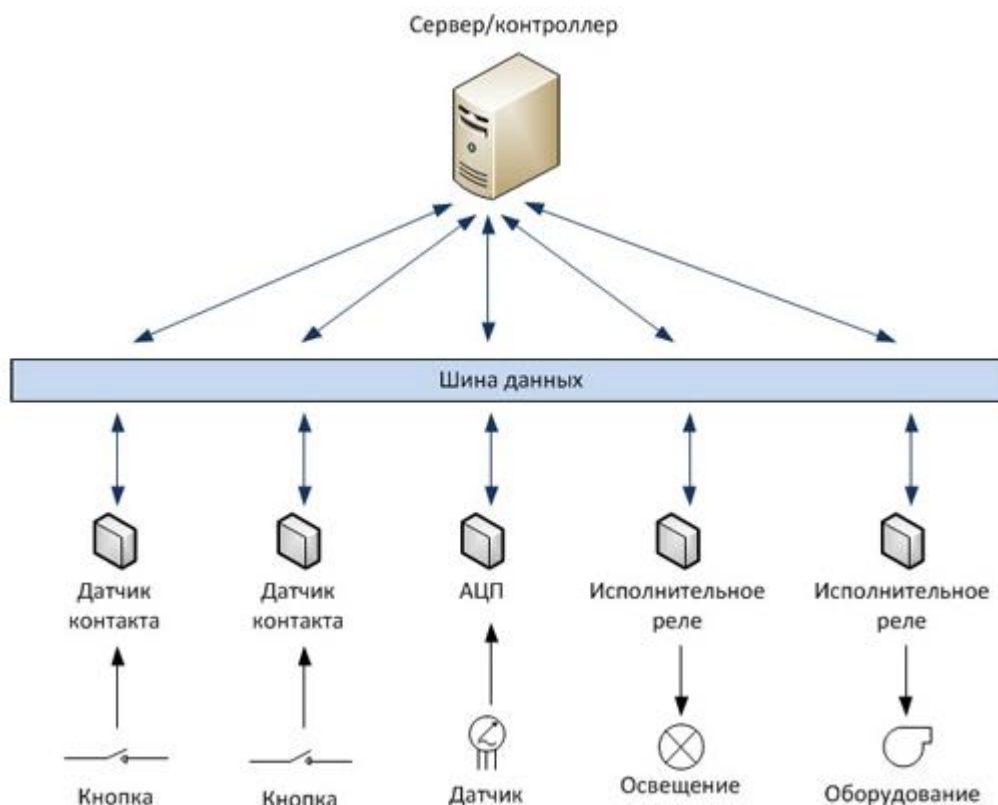
Рис. 34 Схема централизованной системы Умного Дома с главным компьютером
