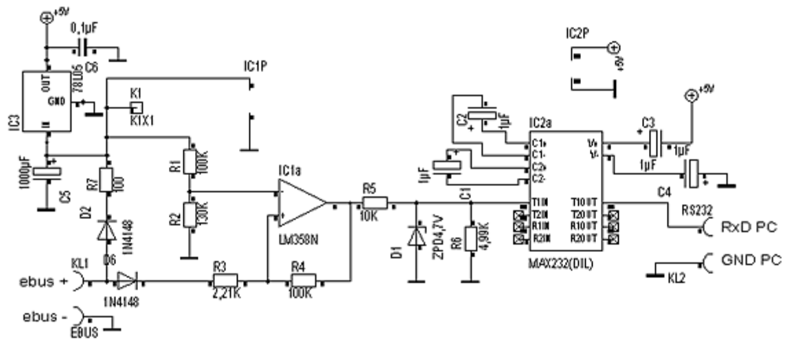
Рис. 65 Принципиальная схема адаптера eBUS-RS232 на базе MAX232
