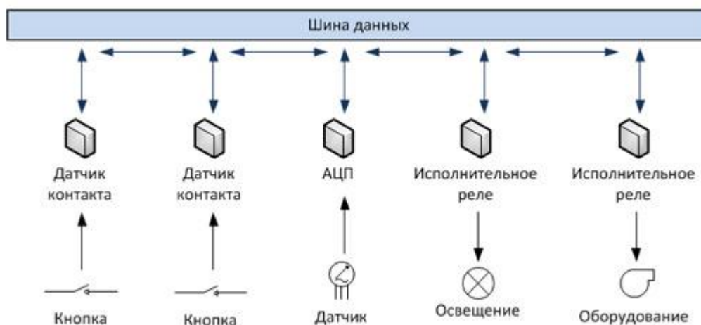
Рис. 33 Схема децентрализованной системы Умного Дома без управляющего контроллера
