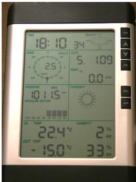
Рис. 75 ЖК-дисплей метеостанции с подключенным USB-кабелем
