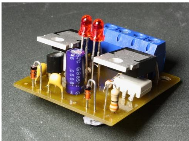
Рис. 50 Плата 2-х канального ключа 1-wire для управления электроприводом 3-х ходового без корпуса.
