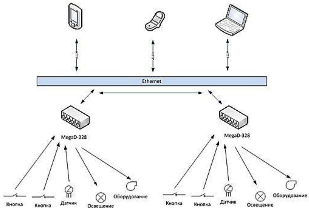
Рис. 35 Схема использования MegaD-328 без сервера. Управление автоматически и через встроенный Web-интерфейс
