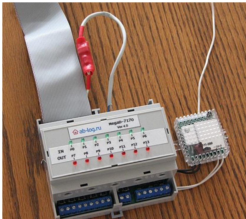
Рис. 18 Интеграция элементов pooLite в общую систему Умного Дома
