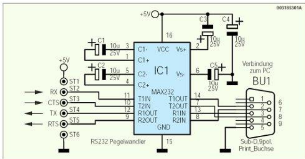
Рис. 56 Схема адаптера TTL-RS232 (MAX232), +5В берем с разъема котла.
