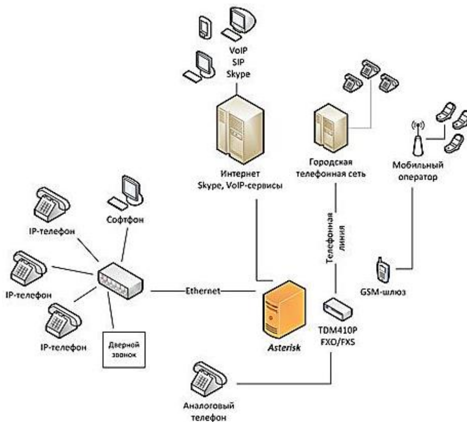
Рис. 89 IP-телефония в доме
