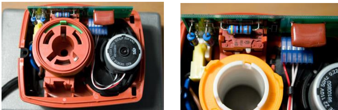
Рис. 47 Устройство термоконтроллера
